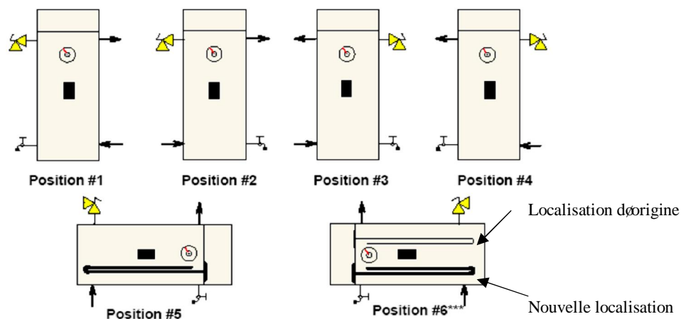
Fig. 2 Positions de montage
