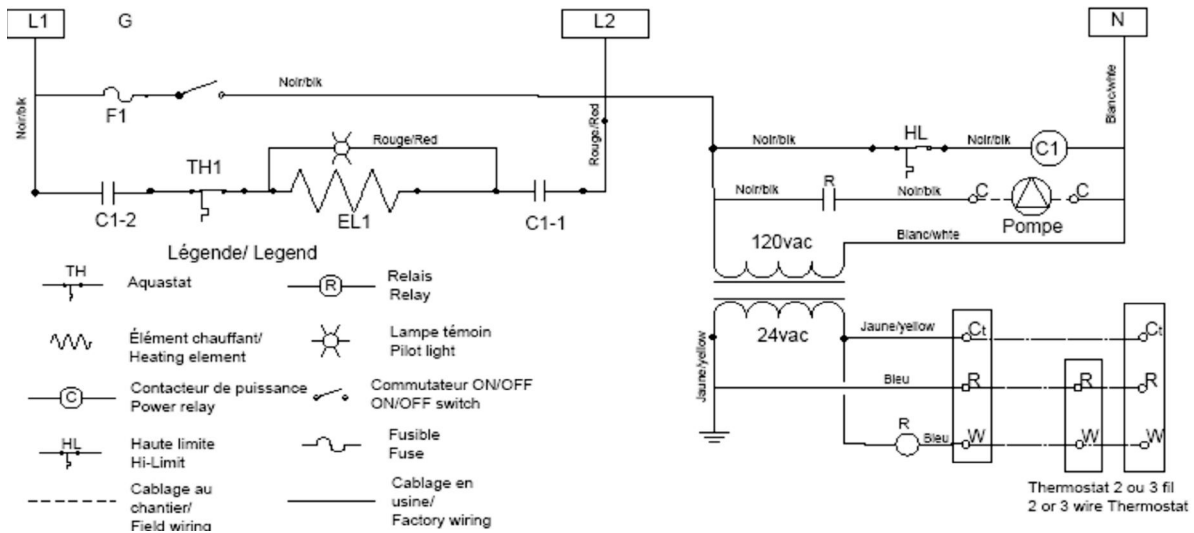
Diagramme électrique/ Wiring diagram BTH MINI 240V 3-6Kw Rev.7/3/11
