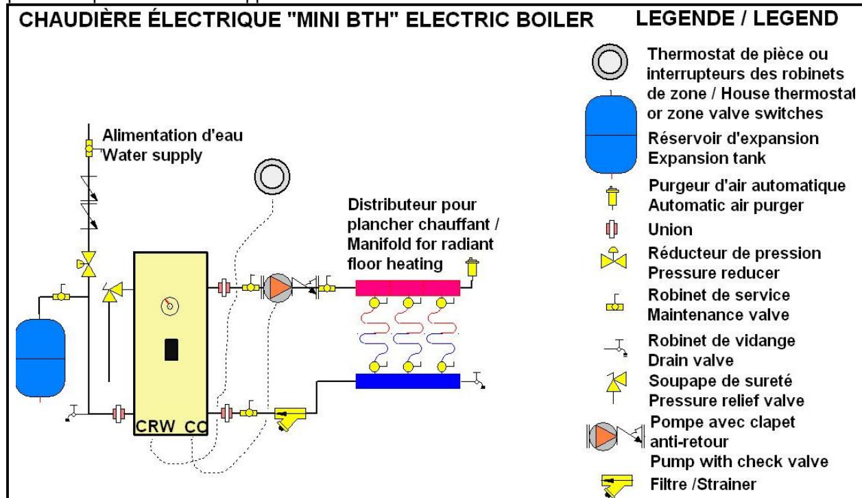
Figure 3 : Schéma d'installation typique
