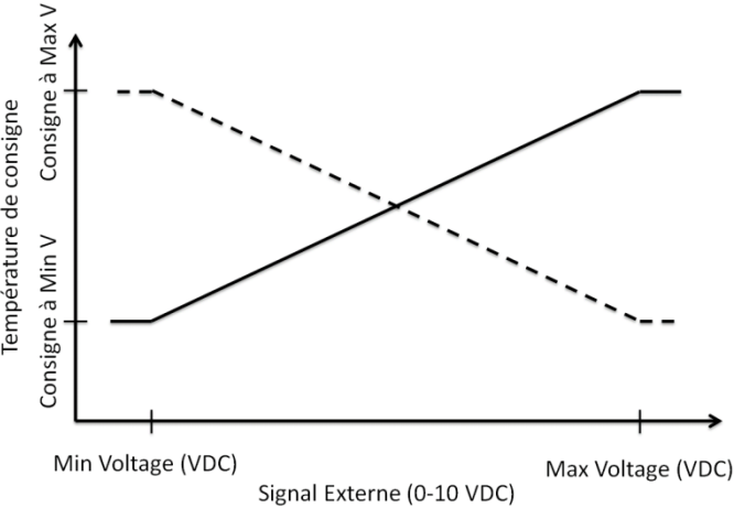
Figure 17 : Courbe d'ajustement DDC 0-10 VDC
