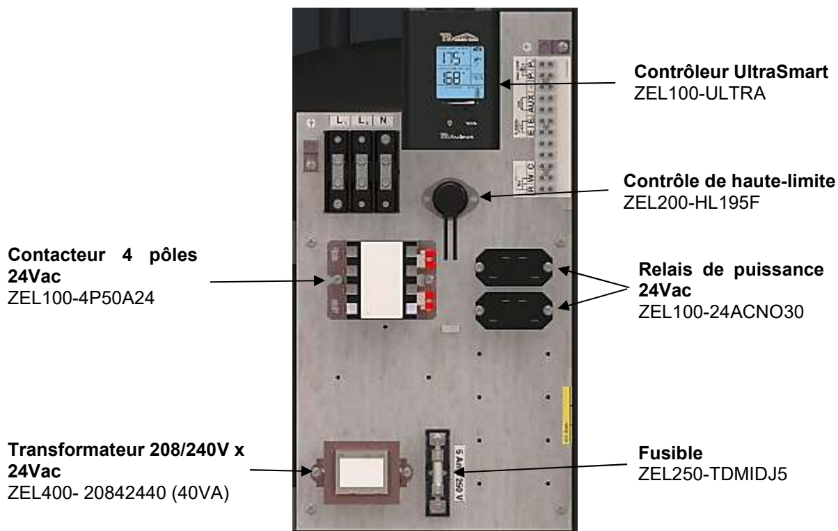
Figure 13: Panneau électrique AltSource 12 kW
