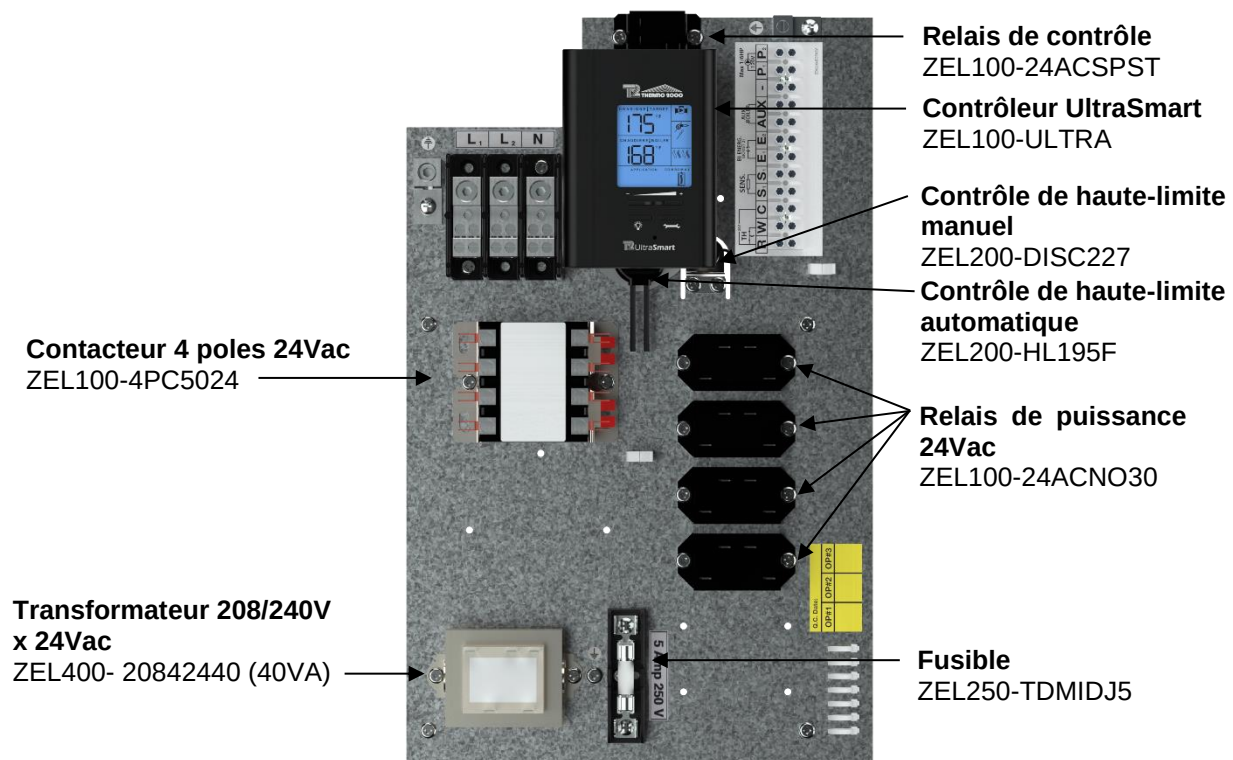
Figure 14: Panneau électrique Altsource 15 à 24 kW
