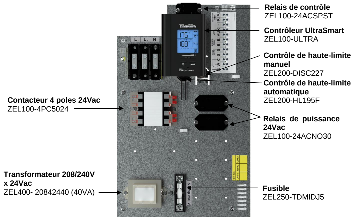
Figure 13: Panneau électrique Altsource 12 kW
