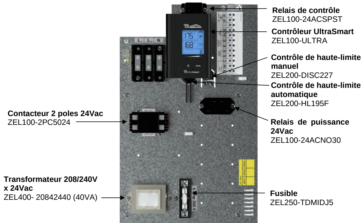
Figure 11: Panneau électrique Altsource 4,5 kW
