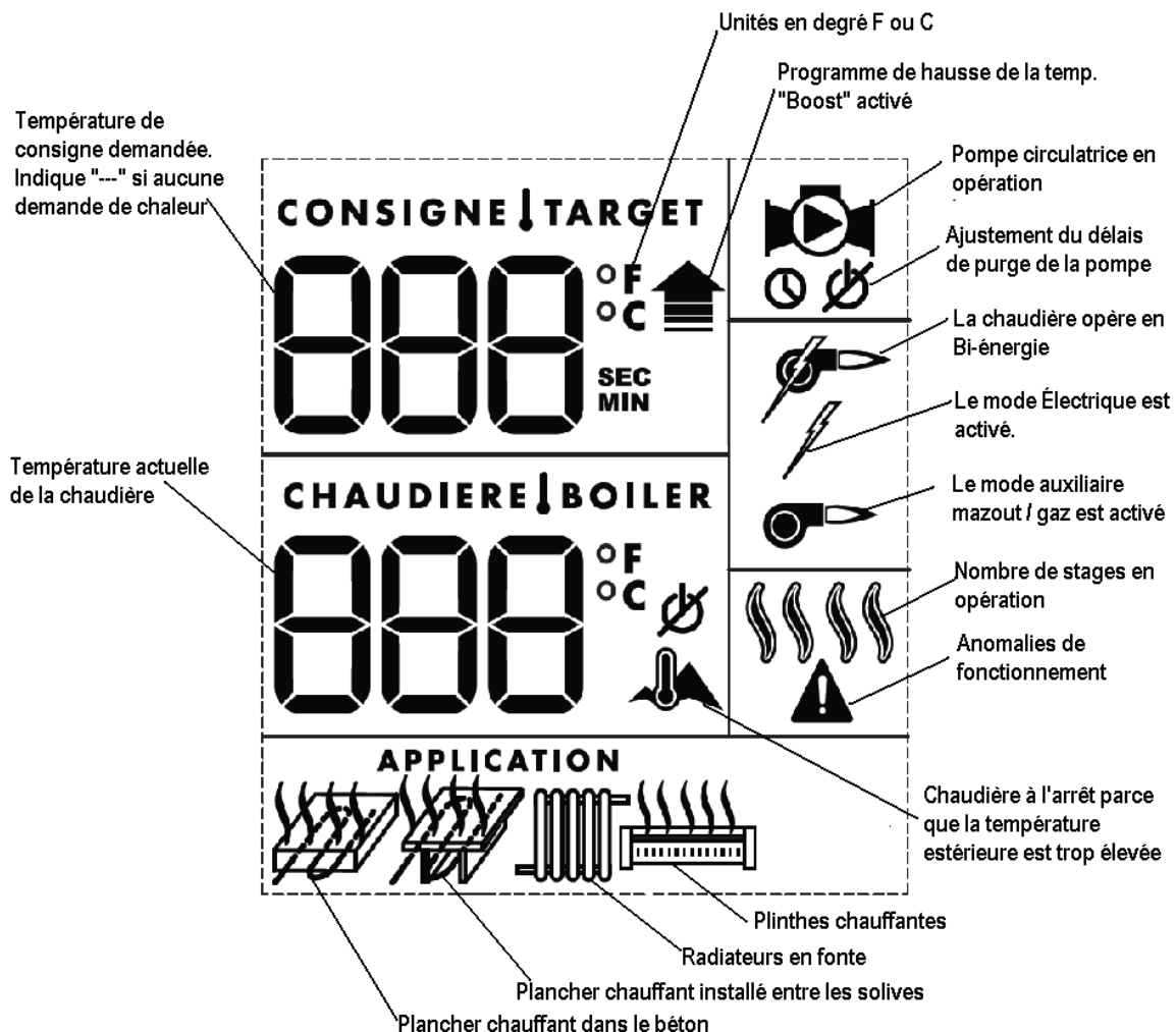
Figure 8 : Interface du contrôleur UltraSmart
