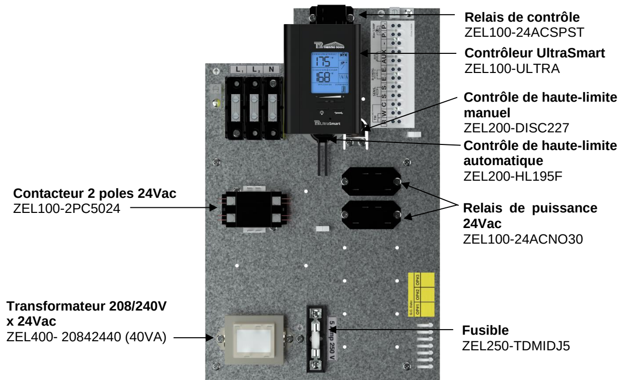
Figure 12: Panneau Électrique Altsource 7,5 et 9 kW
