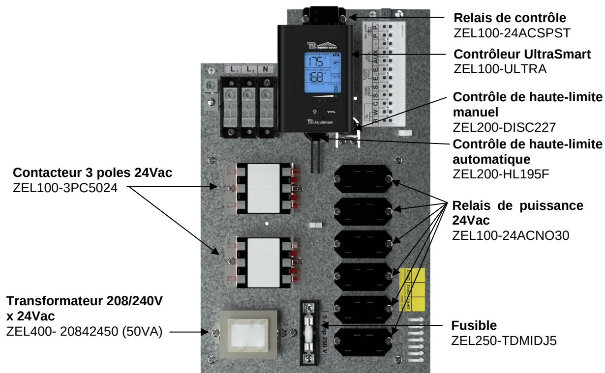
Figure 15: Panneau électrique AltSource 27 et 29 kW
