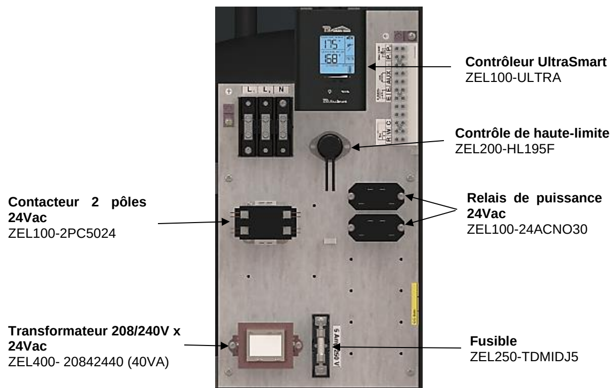
Figure 12: Panneau Électrique AltSource 7,5 et 9 kW
