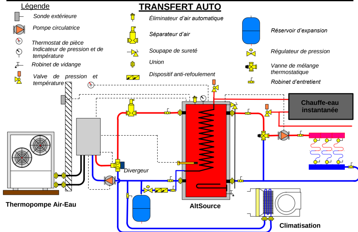
Figure 21 : Schéma d'installation avec thermopompe air-eau pour climatisation et chauffage
