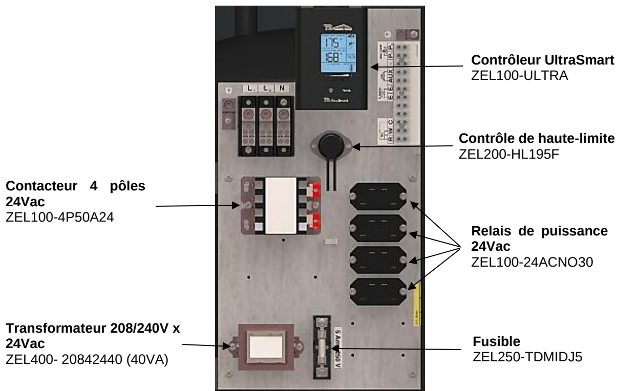
Figure 14: Panneau électrique AltSource 15 à 24 kW
