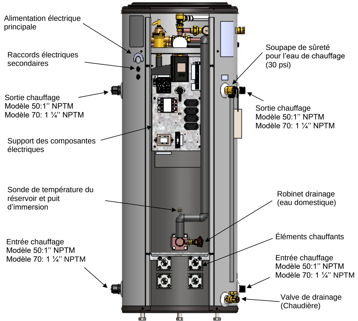
Figure 3: Identification et localisation des composantes du compartiment avant
