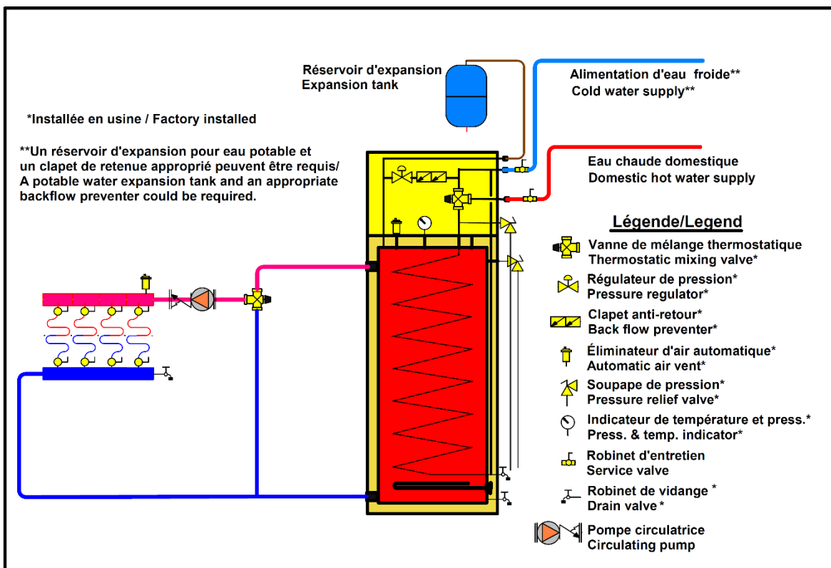
Figure 4: Schéma d'installation de base pour applications avec plancher chauffant
