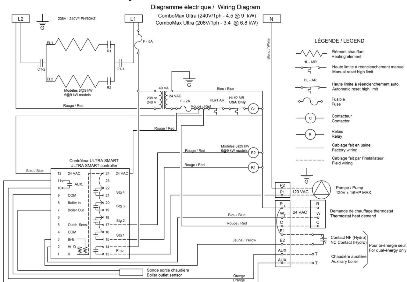
Figure 12: Branchements en bi-énergie
