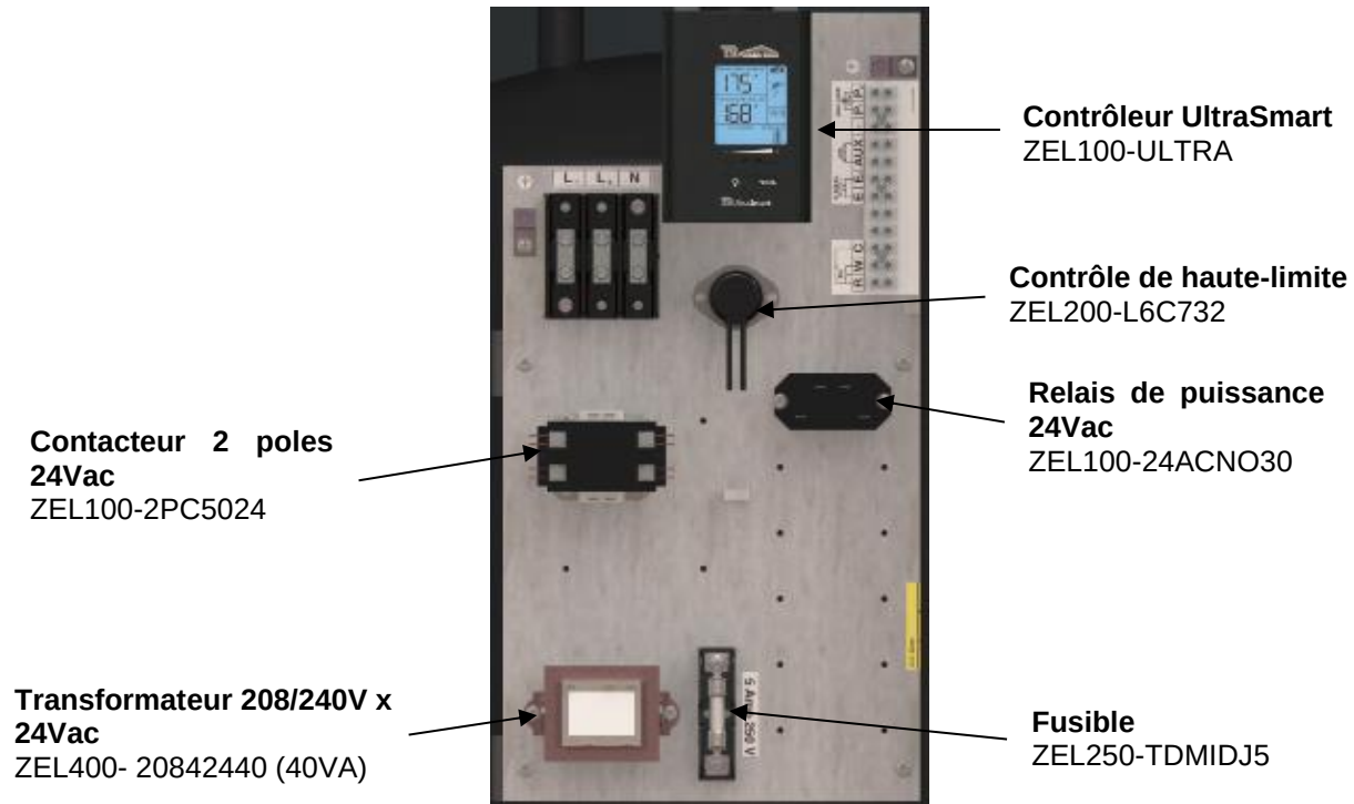
Figure 15: Panneau électrique Combomax Ultra 4,5 kW
