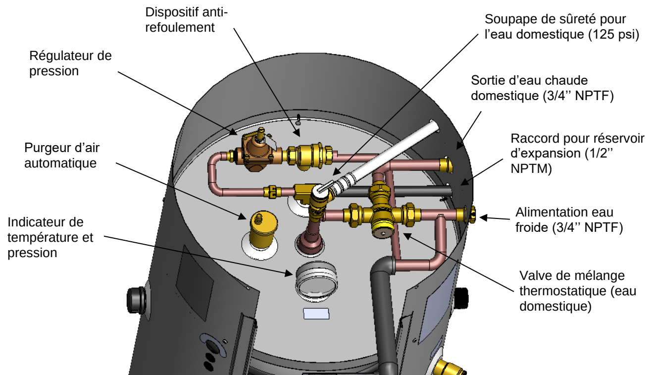
Figure 2: Identification et localisation des composantes du compartiment supérieur
