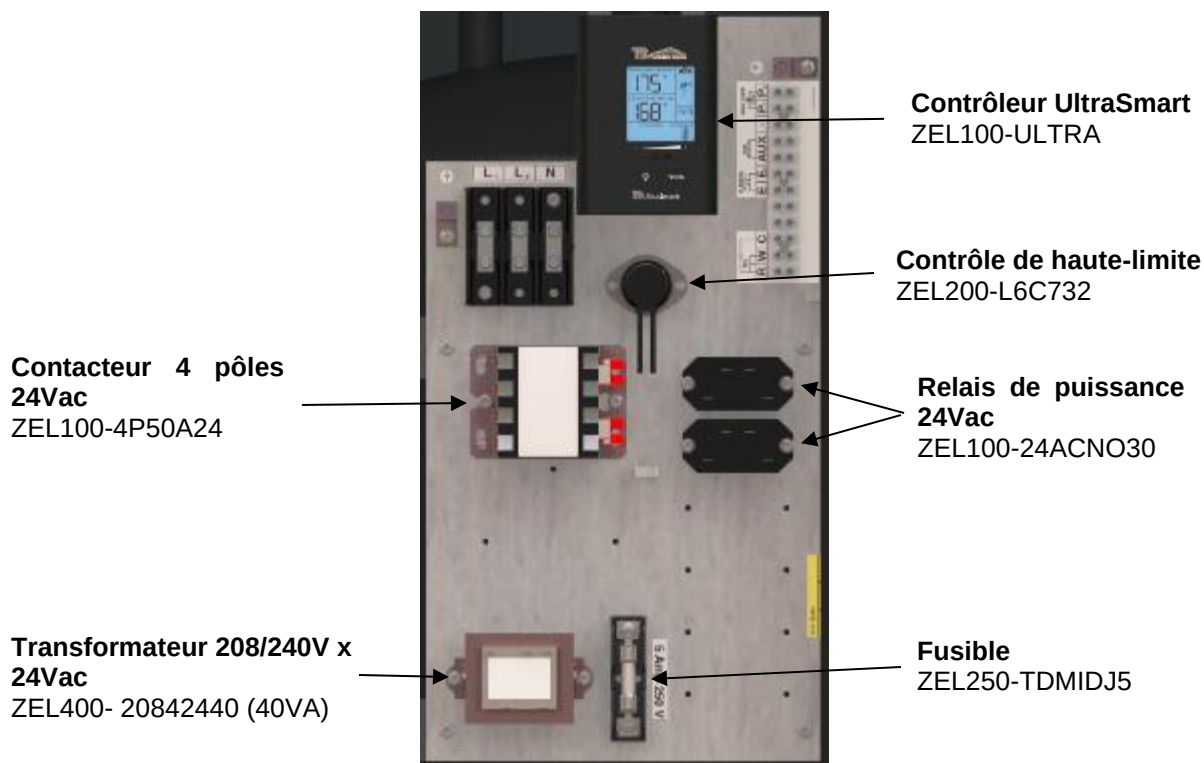
Figure 17: Panneau électrique Combomax Ultra 12 kW
