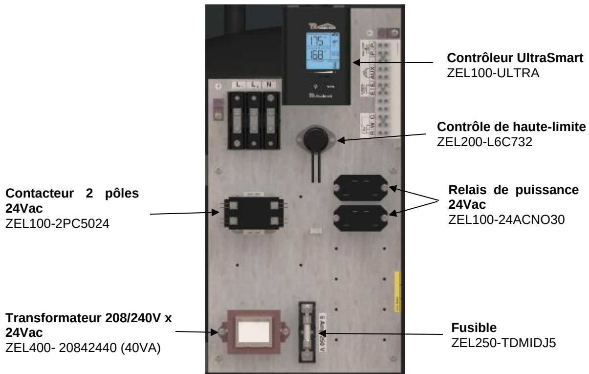
Figure 16: Panneau Électrique Combomax Ultra 7,5 et 9 kW
