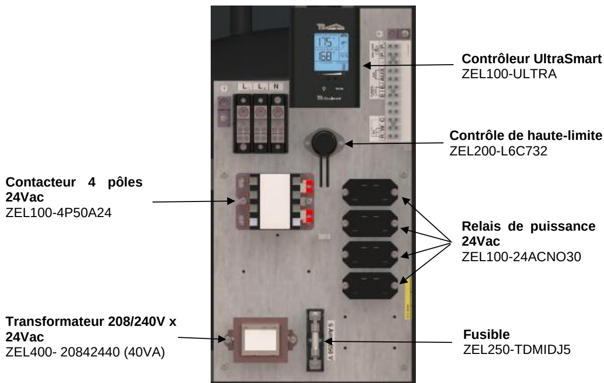
Figure 18: Panneau électrique Combomax Ultra 15 à 24 kW
