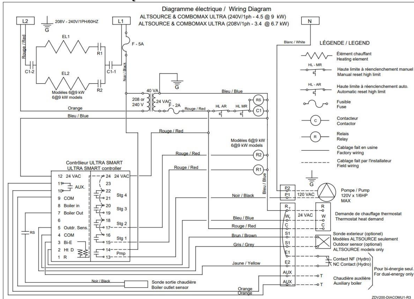
Figure 12: Branchements en bi-énergie
