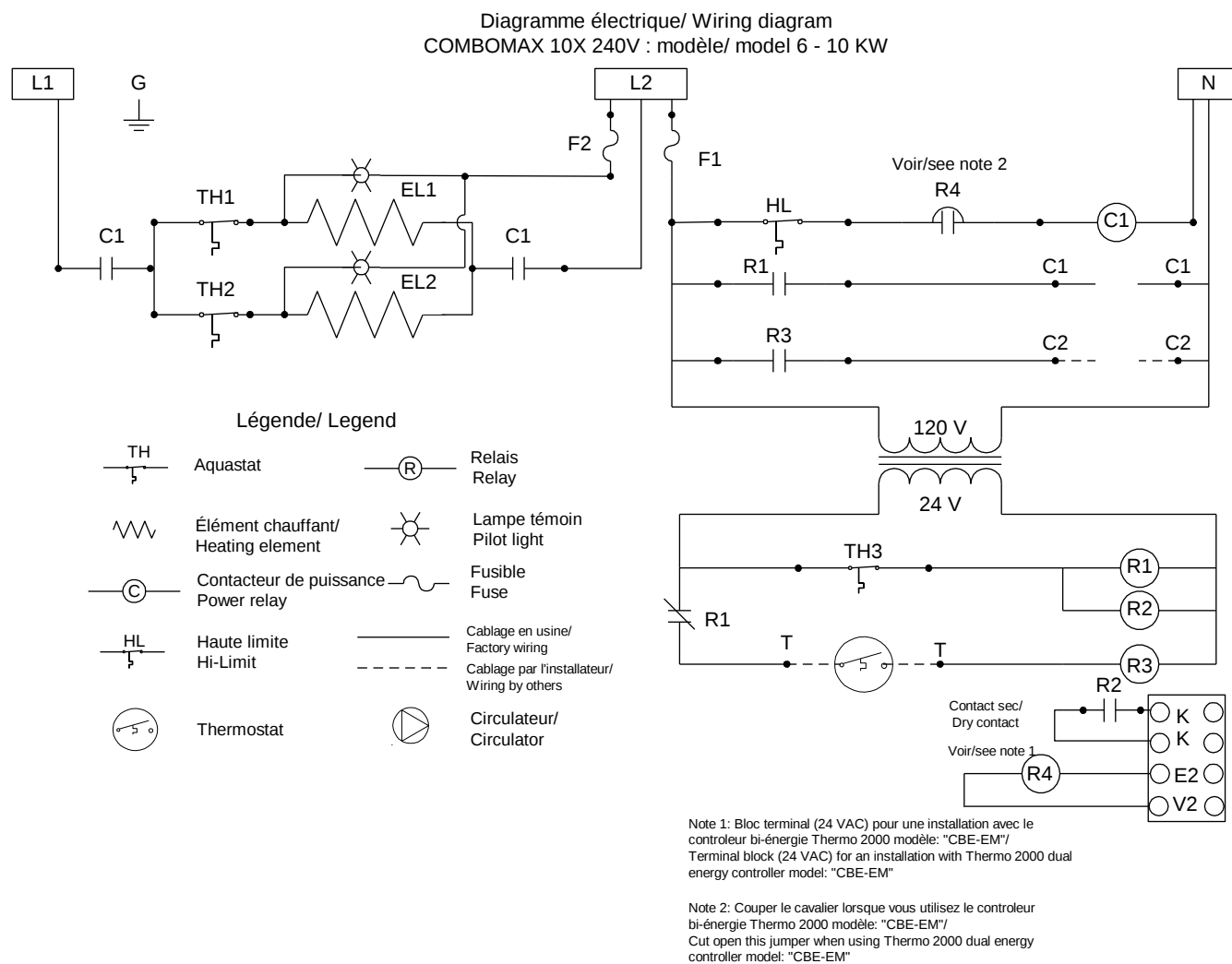
Figure 4 : Schéma électrique 240V 6-10 kW
