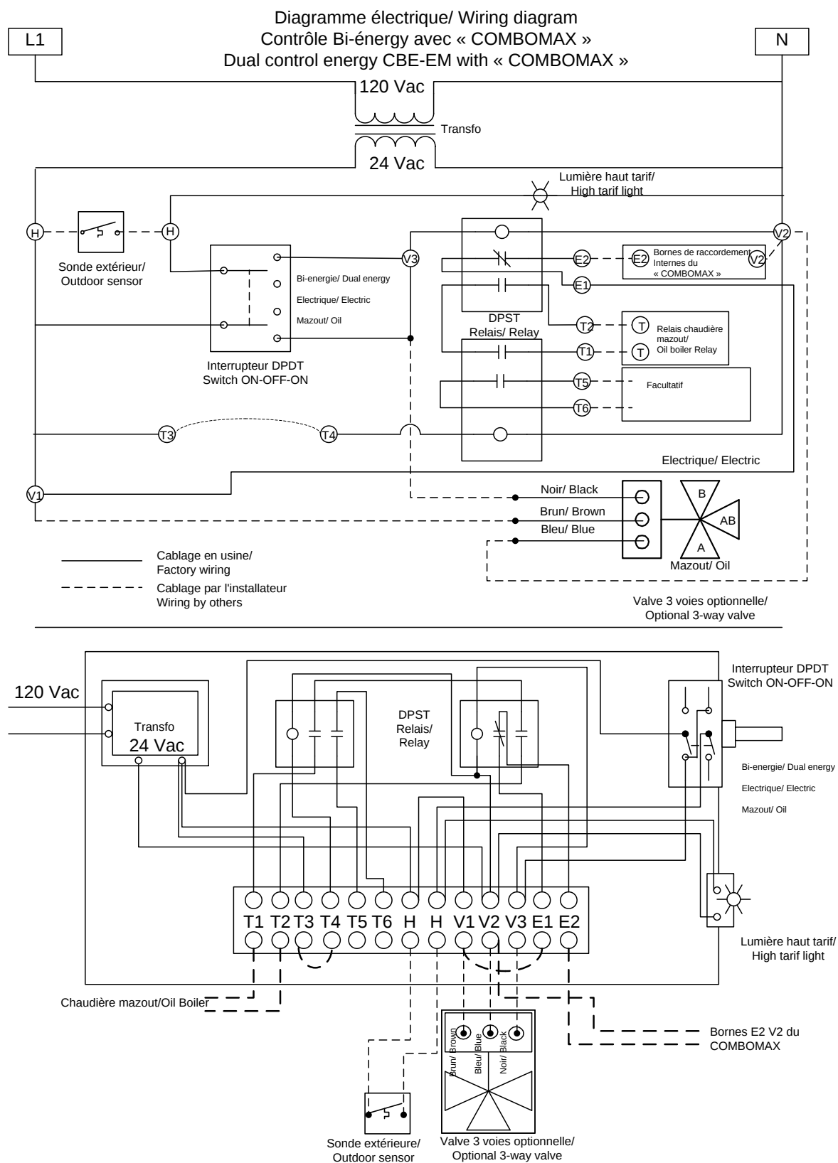
Figure 9: Schéma électrique bi-énergie
