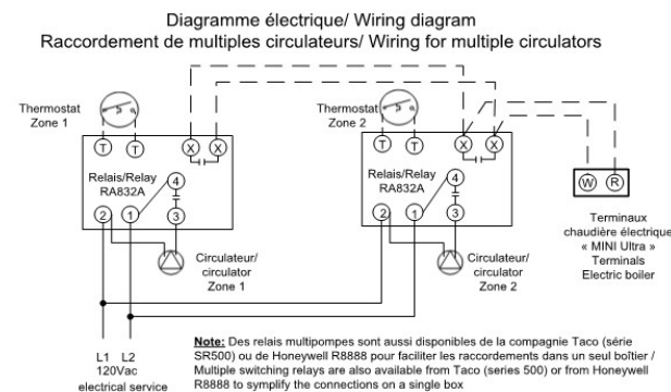
Figure 11 : Schéma de zonage par pompes multiples
