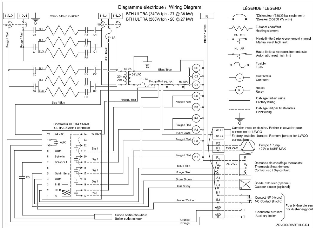
Figure 16 : Diagramme électrique (27-36 KW)
