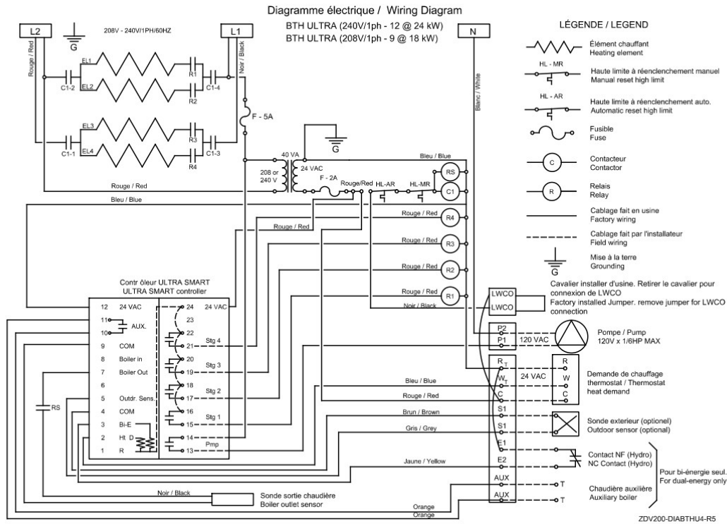
Figure 16 : Diagramme électrique (12-24 KW)
