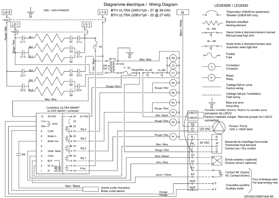
Figure 17 : Diagramme électrique (27-36 KW)
