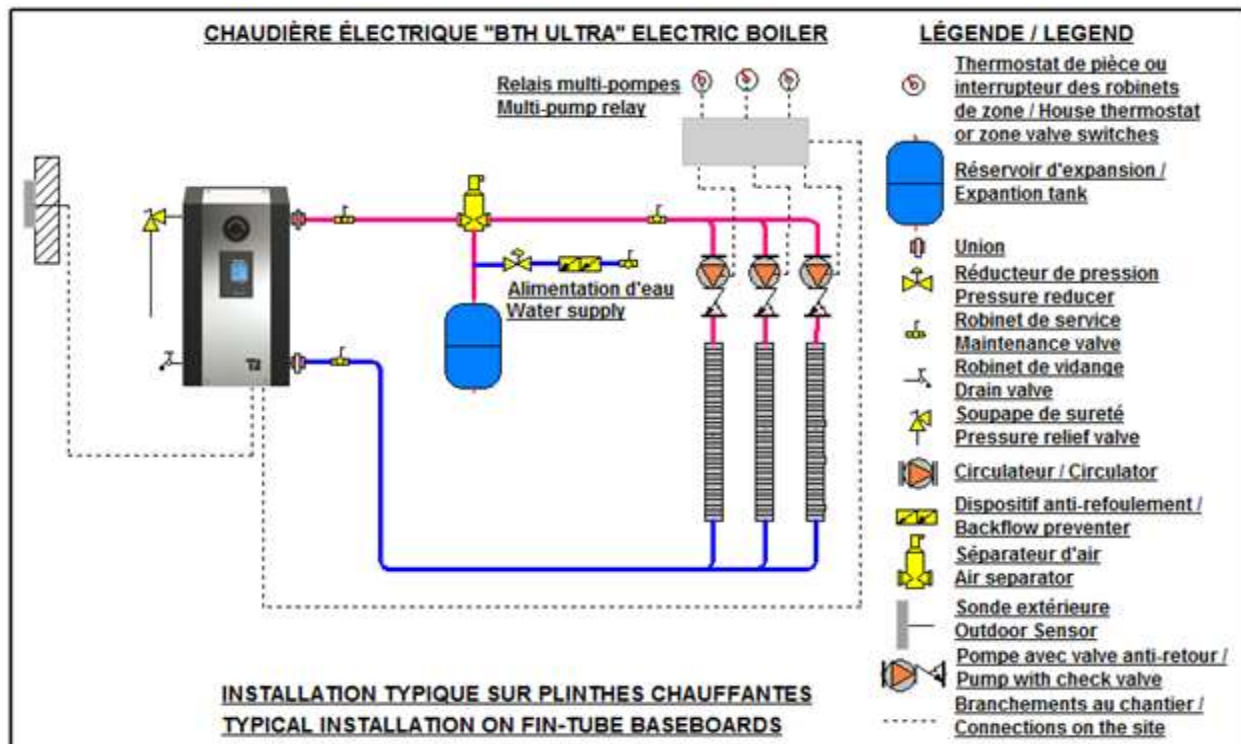
Figure 7 : Installation typique pour une configuration multi-pompes
