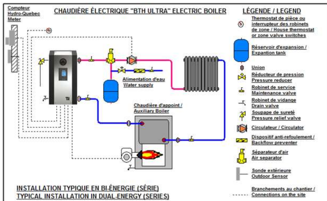
Figure 8 : Installation typique pour une configuration bi-énergie en série
