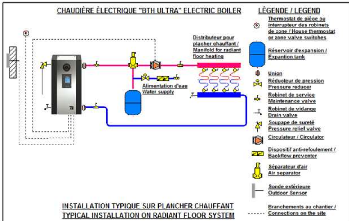
Figure 5 : Installation typique sur système de plancher chauffant
