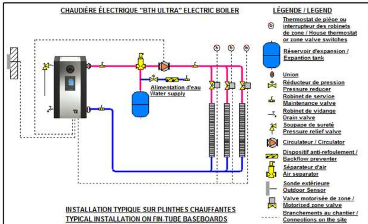
Figure 6 : Installation typique avec plinthes chauffantes et valves de zonage
