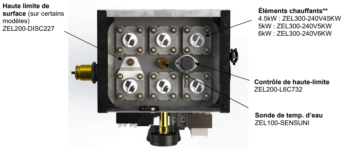
Figure 23 : Pièces de rechange, vue de dessus (27à36 KW)
