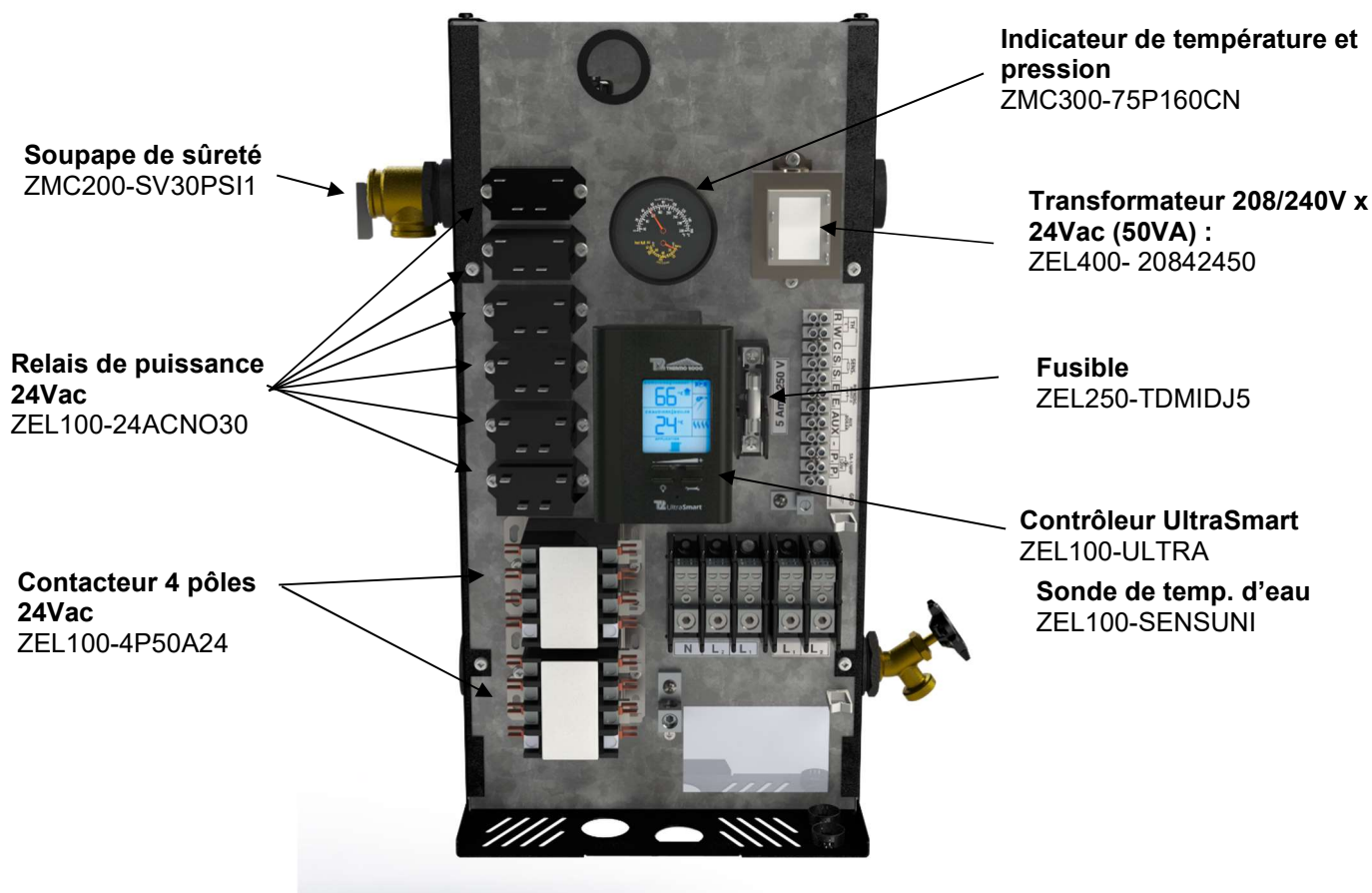
Figure 22 : Pièces de rechange, vue de face (27-29 KW)
