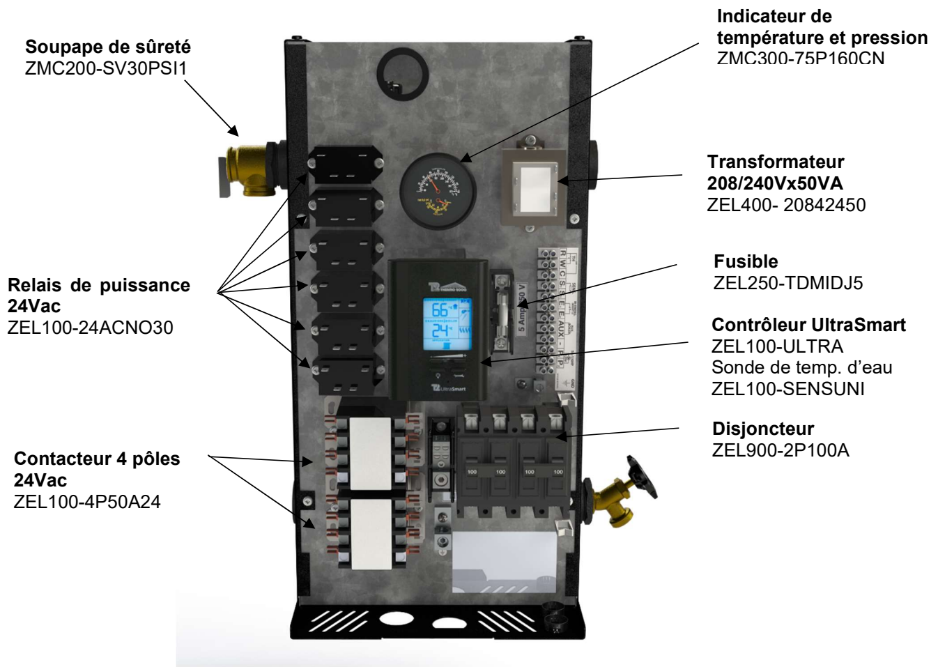
Figure 24 : Pièces de rechange, vue de face (33-36 KW)
