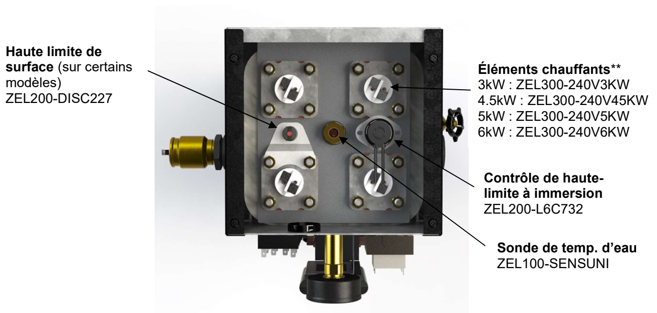
Figure 21 : Pièces de rechange, vue de dessus (12-24 KW)
