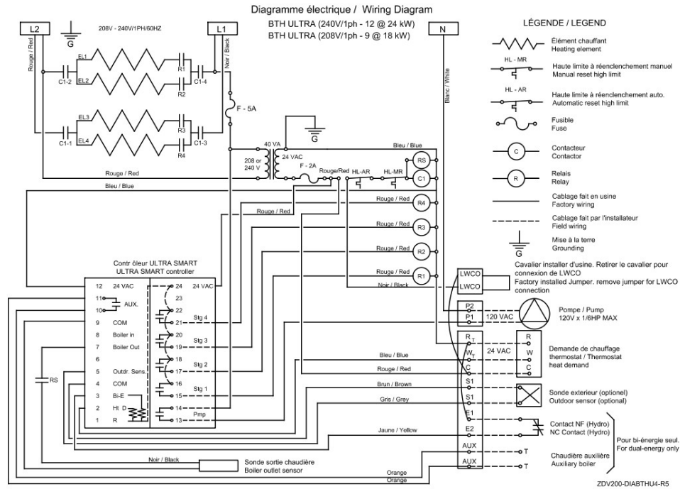
Figure 16 : Diagramme électrique (12-24 KW)
