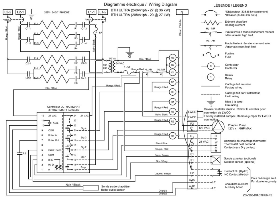
Figure 17 : Diagramme électrique (27-36 KW)
