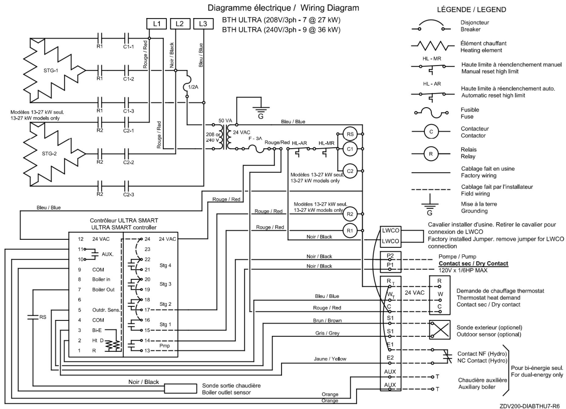
Figure 15 : Diagramme électrique 208/240V-3ph
