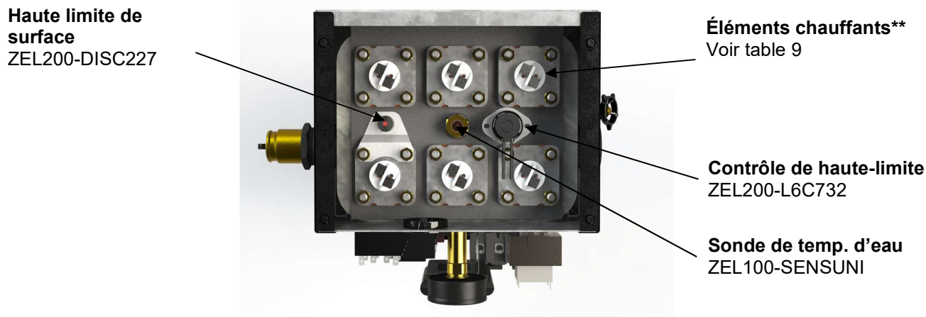
Figure 23 : Pièces de rechange, BTH Ultra 208/240/480/600V-3 ph.
