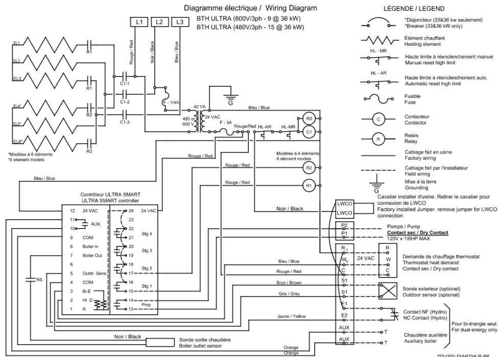
Figure 16 : Diagramme électrique 480/600V-3ph
