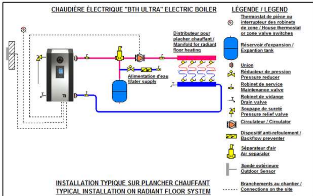
Figure 4 : Installation typique sur système de plancher chauffant
