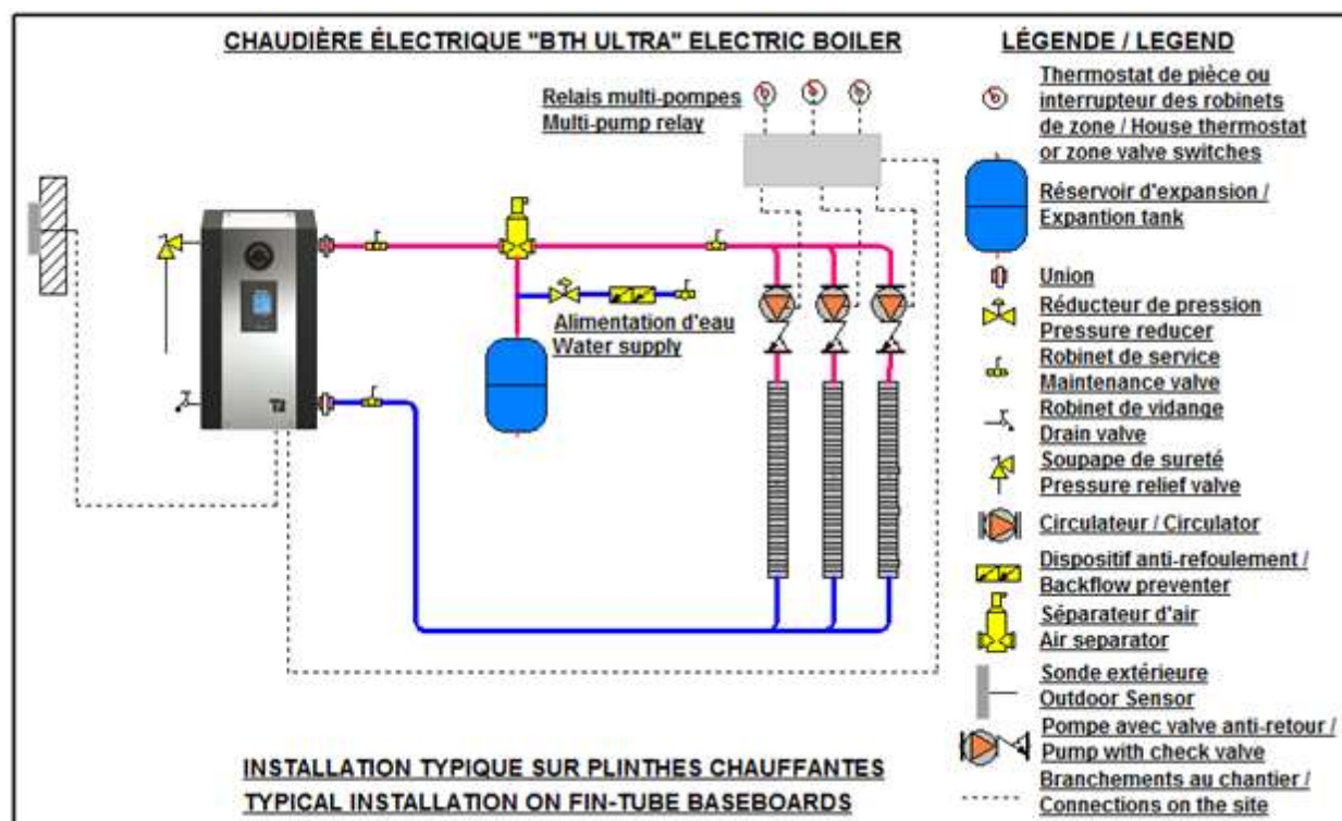
Figure 6 : Installation typique pour une configuration multi-pompes
