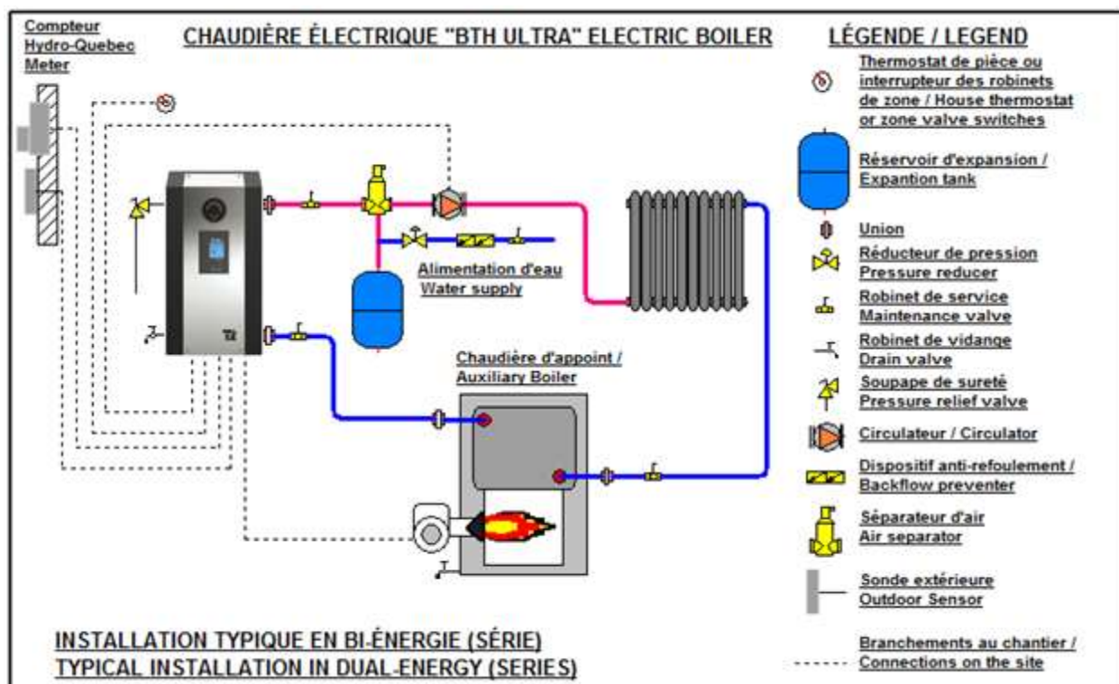
Figure 7 : Installation typique pour une configuration bi-énergie en série
