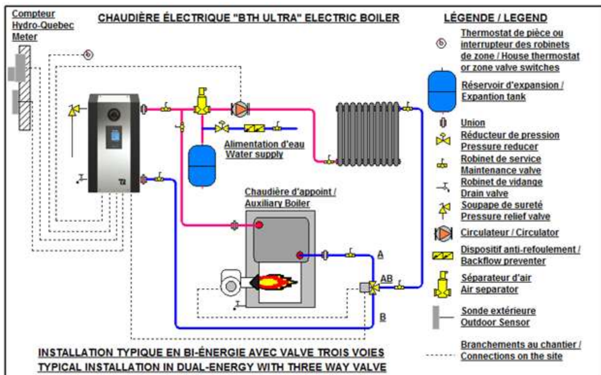
Figure 8 : Installation typique pour une configuration bi-énergie avec valve 3 voies
