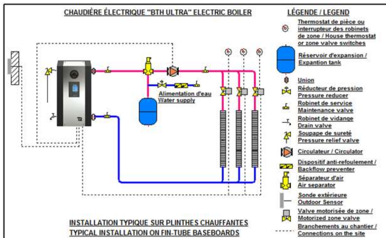
Figure 5 : Installation typique avec plinthes chauffantes et valves de zonage
