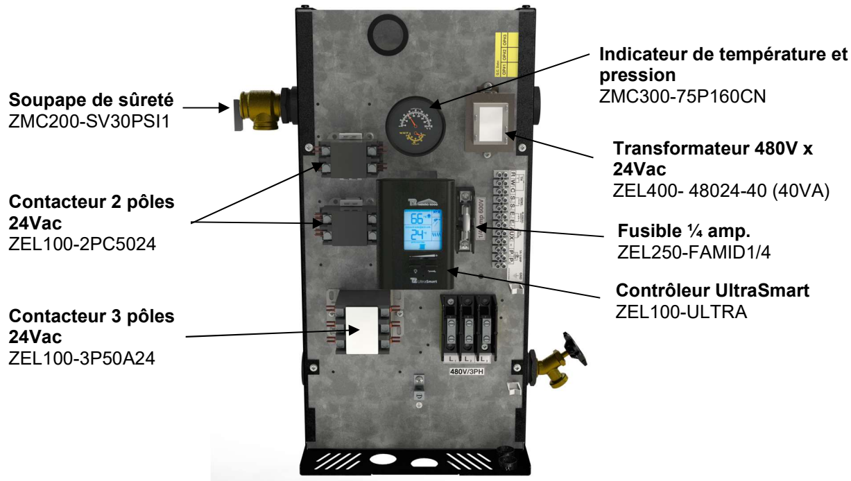
Figure 21 : Pièces de rechange BTH Ultra 480V-3 ph.
