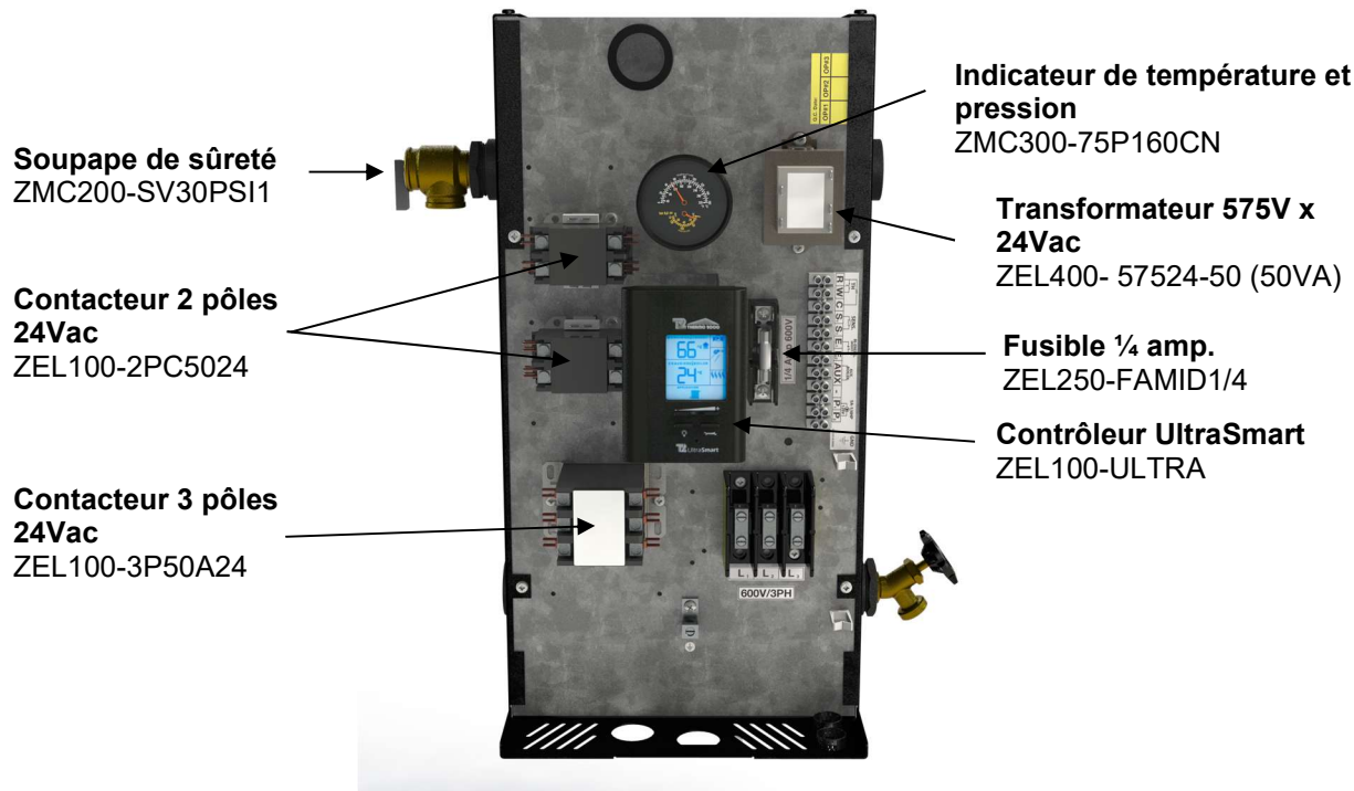
Figure 22 : Pièces de rechange BTH Ultra 600V-3 ph.
