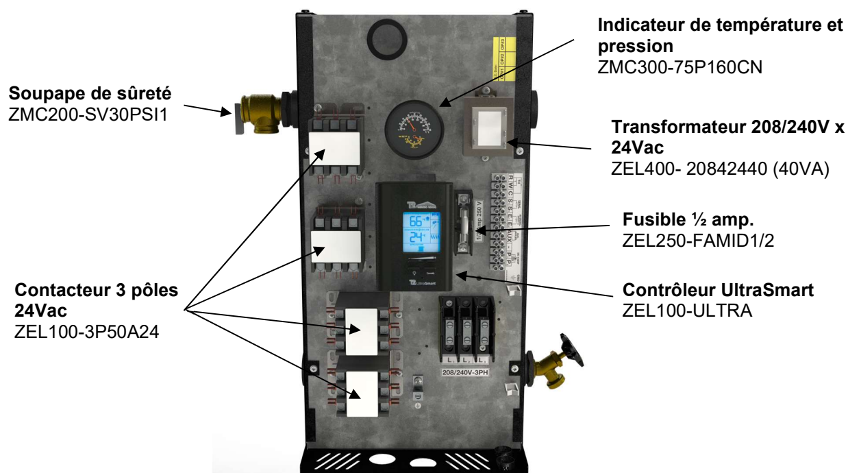
Figure 20 : Pièces de rechange BTH Ultra 208/240V-3 ph.
