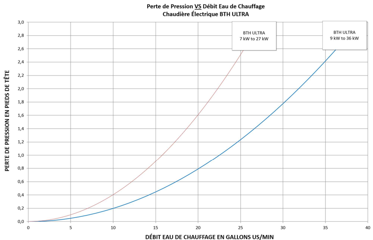
Figure 3 : Diagramme de perte charge
