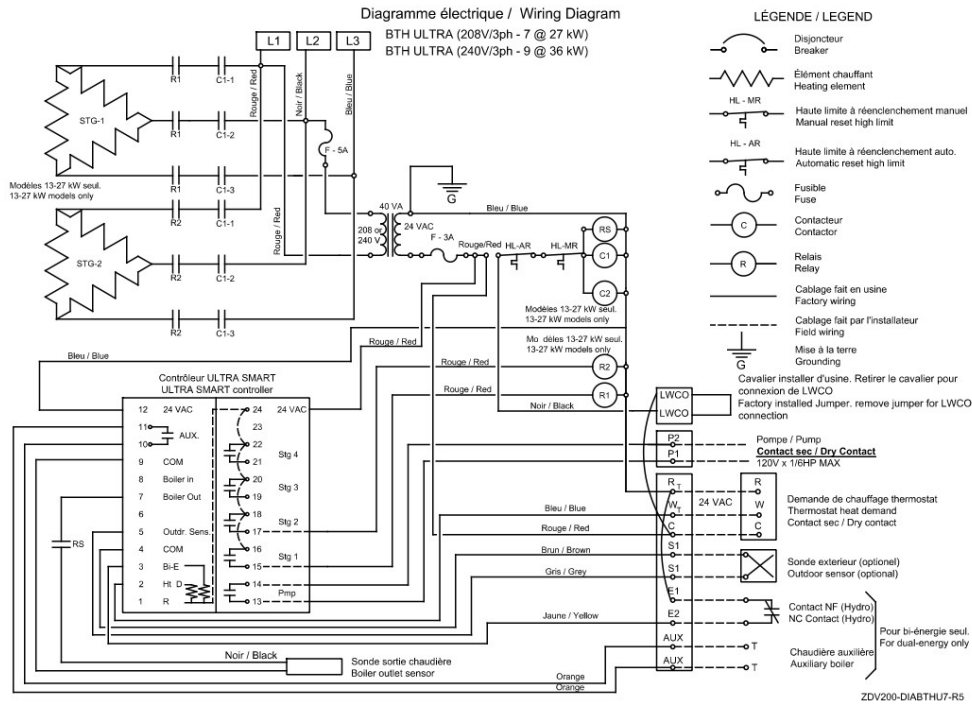
Figure 15 : Diagramme électrique 208/240V-3ph
