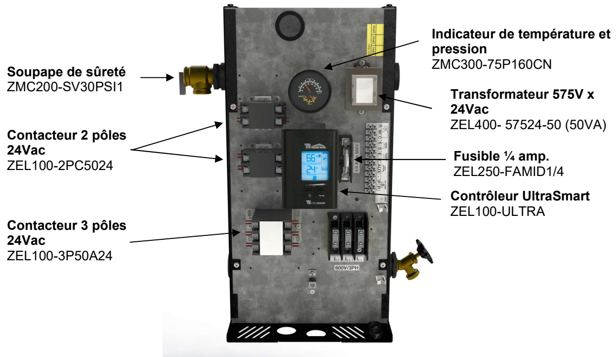
Figure 22 : Pièces de rechange BTH Ultra 600V-3 ph.
