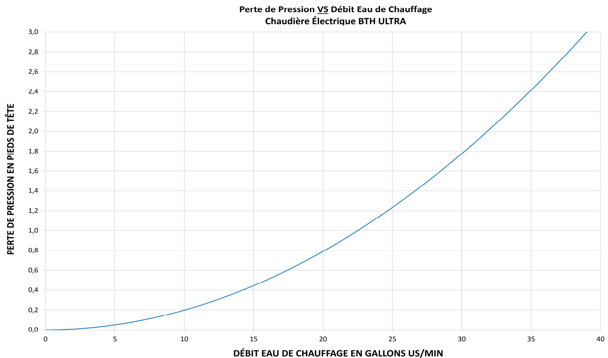
Figure 3 : Diagramme de perte charge
