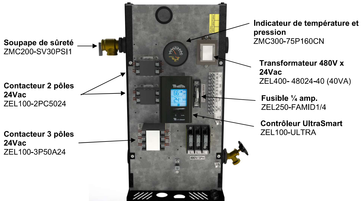
Figure 20 : Pièces de rechange BTH Ultra 480V-3 ph.
