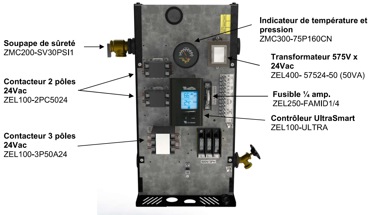
Figure 21 : Pièces de rechange BTH Ultra 600V-3 ph.
