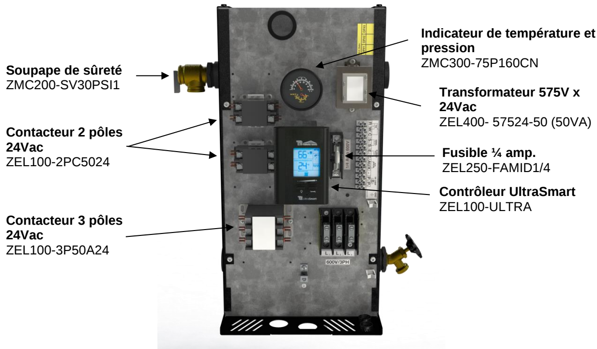
Figure 19 : Pièces de rechange BTH Ultra 600V-3 ph.
