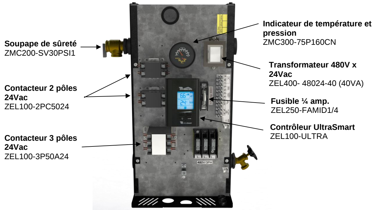
Figure 18 : Pièces de rechange BTH Ultra 480V-3 ph.
