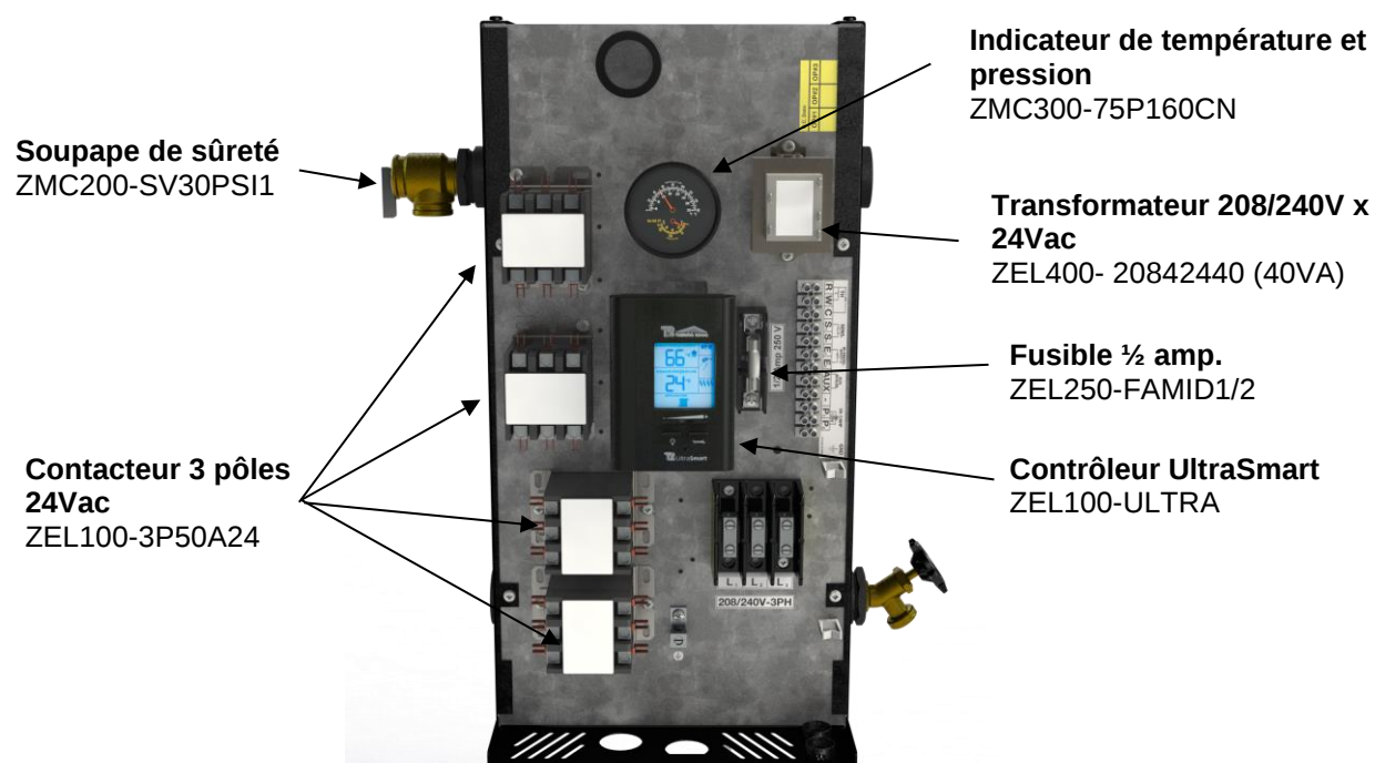
Figure 17 : Pièces de rechange BTH Ultra 208/240V-3 ph.
