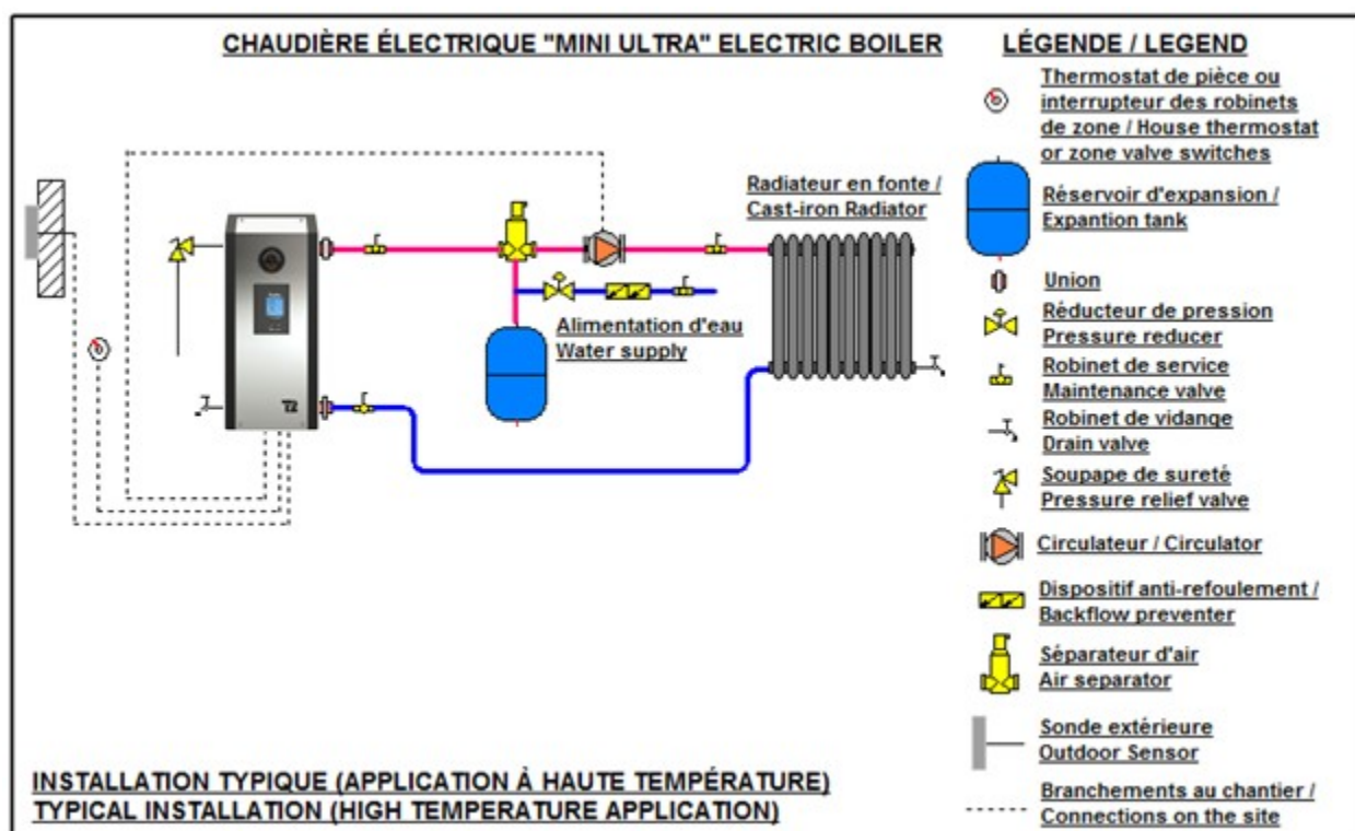
Figure 5 : Schéma d'installation pour application à haute température
