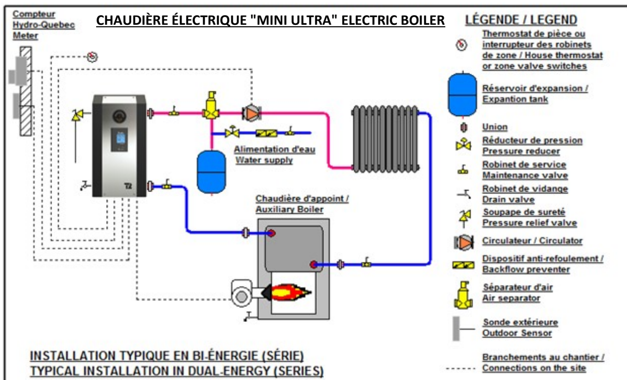
Figure 6 : Installation Bi-énergie en série (modèles USA seulement)
