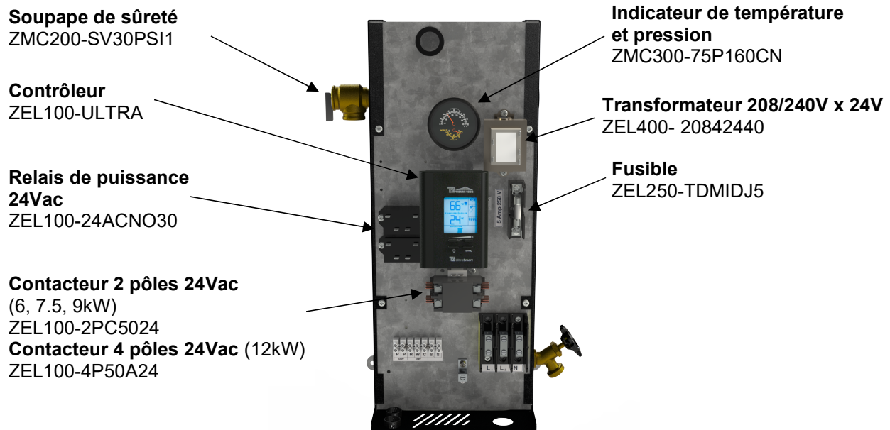
Figure 16 : Pièces de remplacement (Face)
