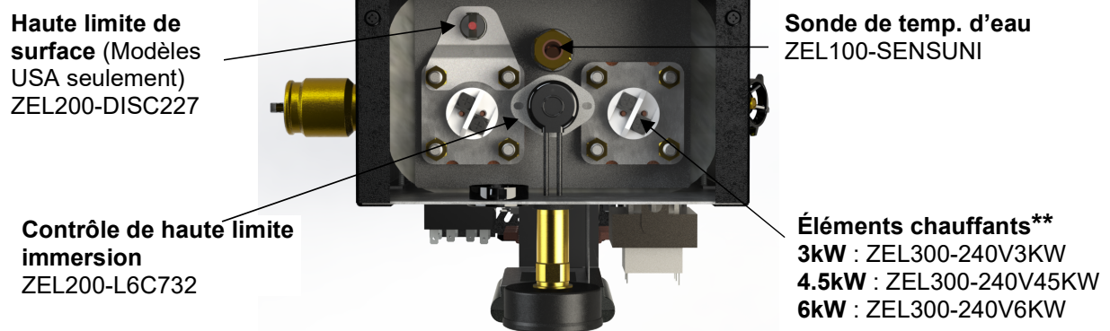
Figure 17 : Pièces de remplacement (Dessus)
