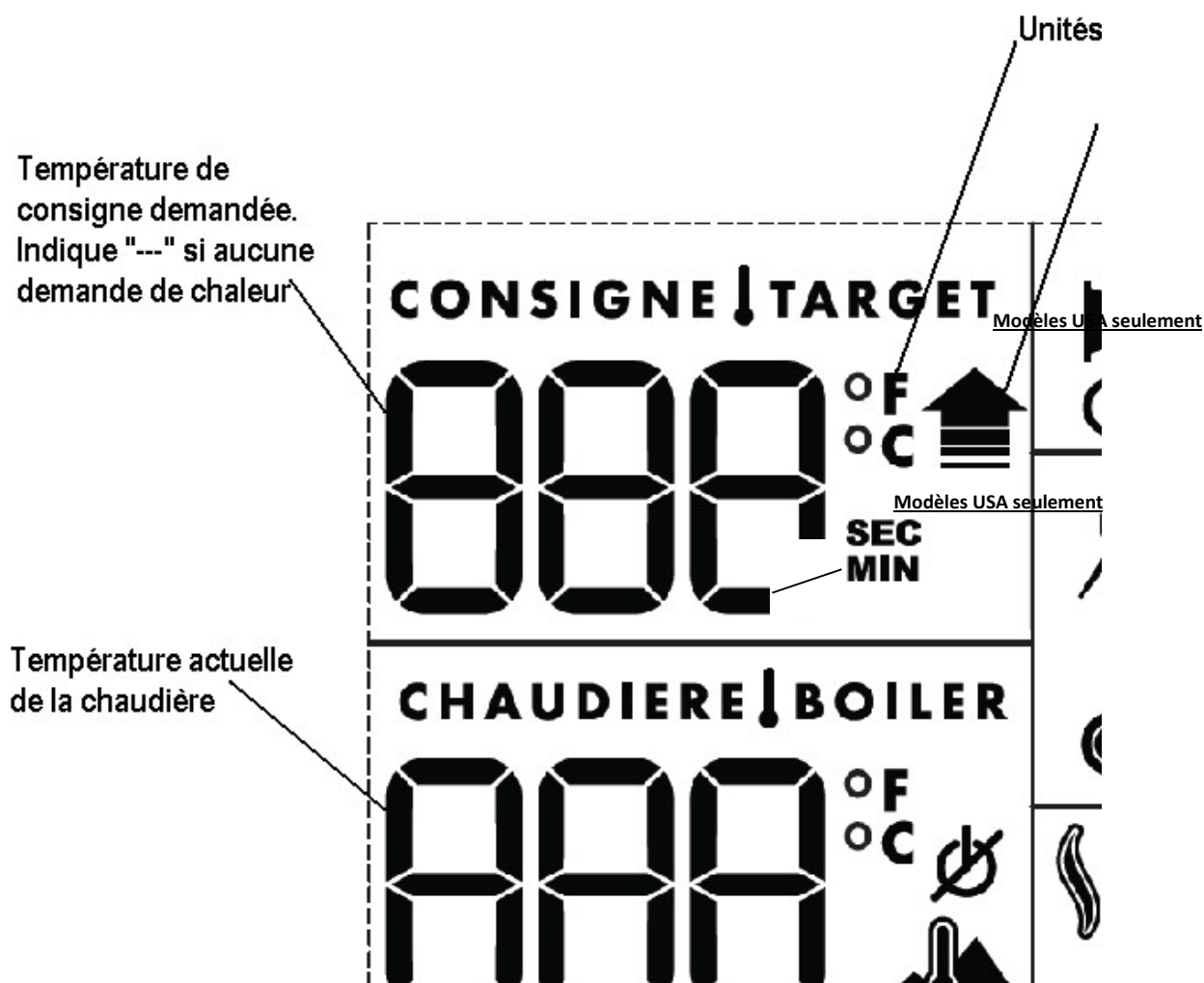
Figure 13 : Affichage du contrôleur UltraSmart
