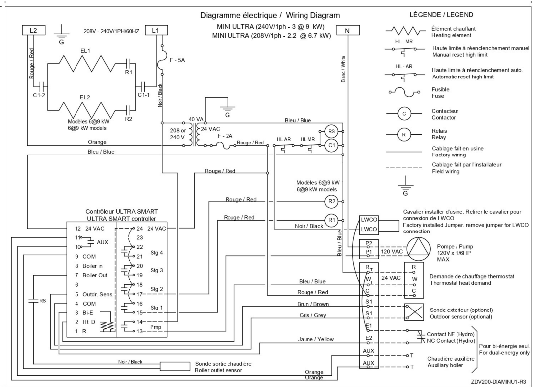
Figure 11 : Diagramme électrique (3-9 KW)
