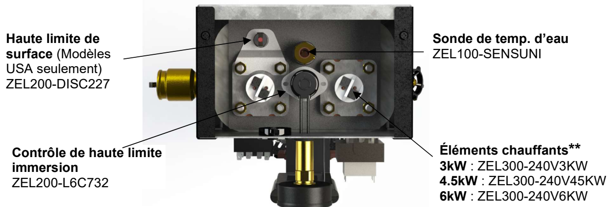
Figure 18 : Pièces de remplacement (Dessus)
