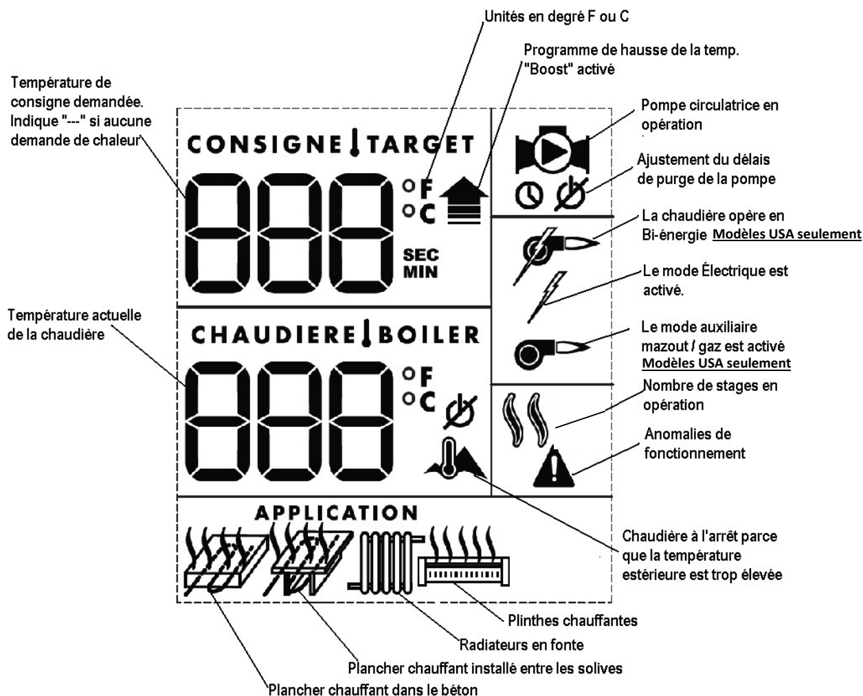
Figure 14 : Affichage du contrôleur UltraSmart
