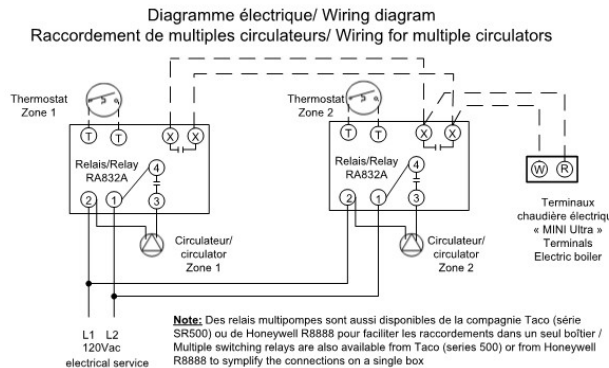
Figure 8 : Schéma de zonage par pompes multiples
