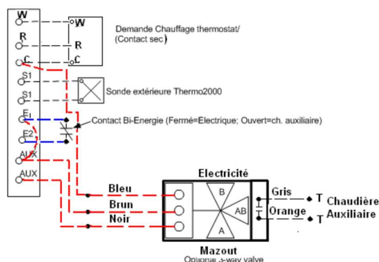
Figure 11 : Raccord avec valve trois voies
