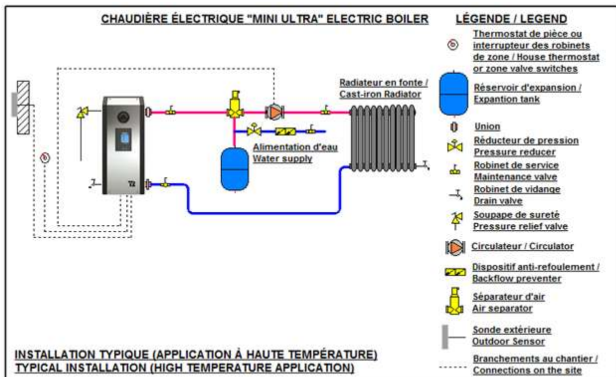
Figure 5 : Sch  ma d'installation pour application    haute temp  rature
