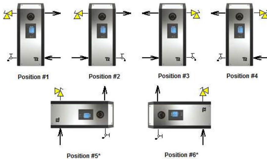
Figure 2 : Position de montage
