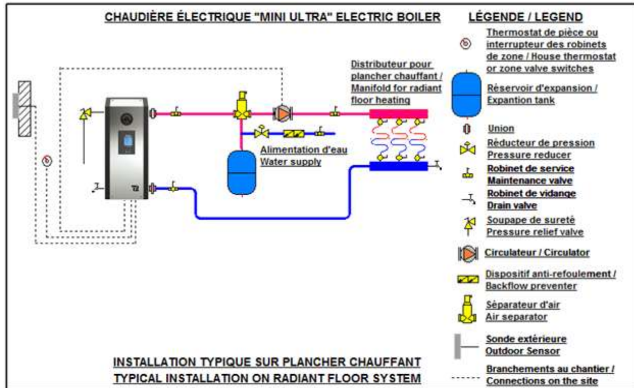
Figure 4 : schéma d'installation sur plancher chauffant
