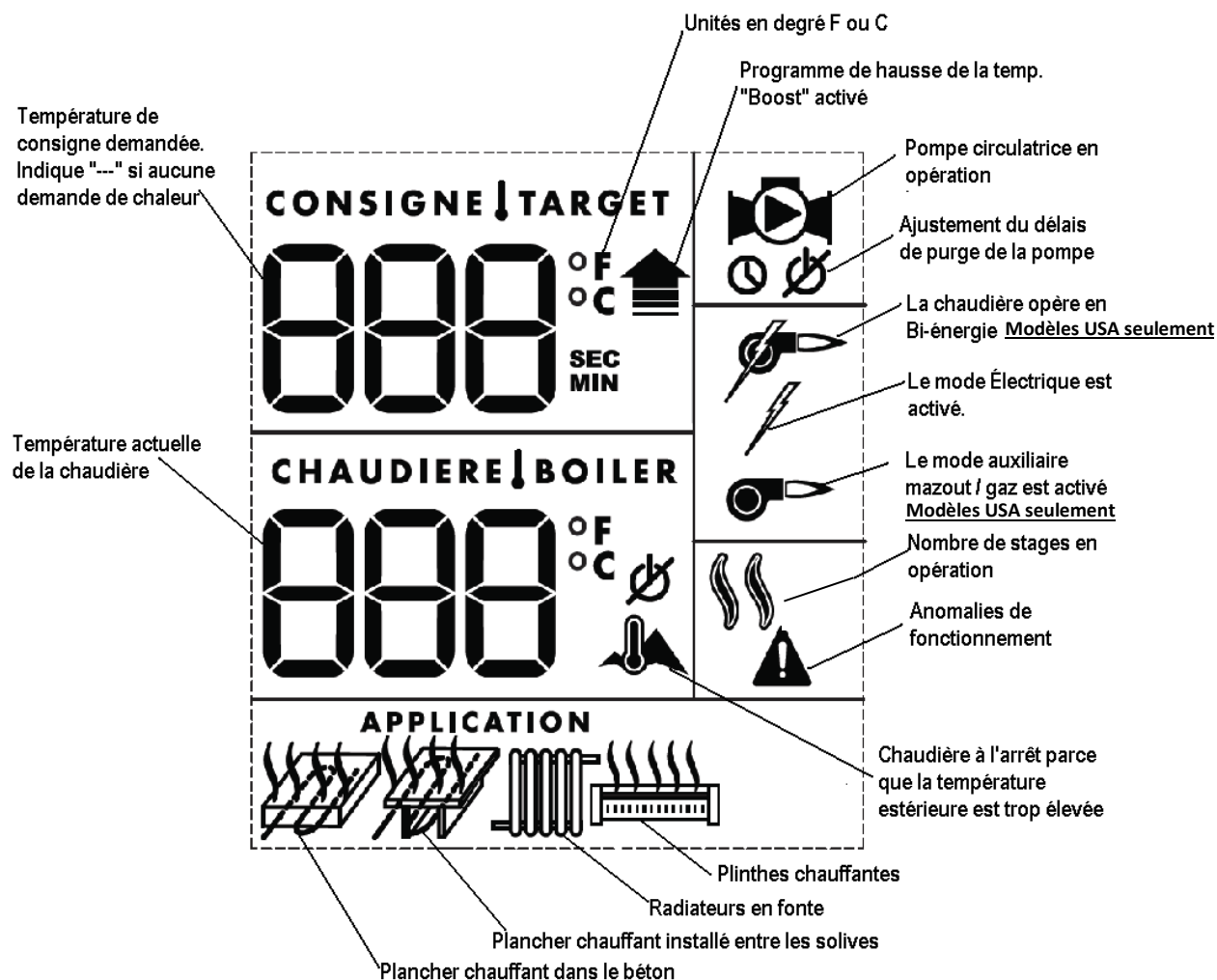
Figure 12 : Affichage du contrôleur UltraSmart
