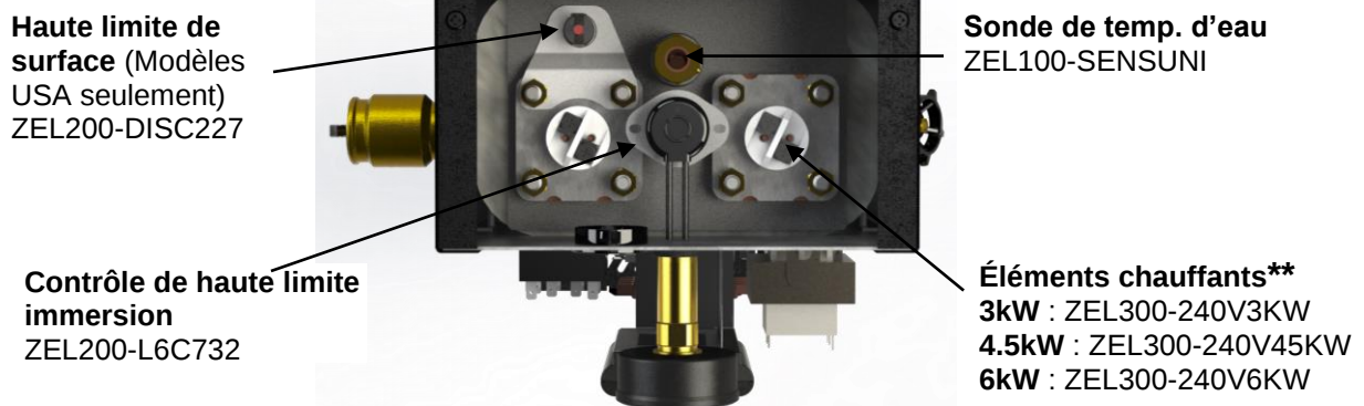
Figure 16 : Pièces de remplacement (Dessus)
