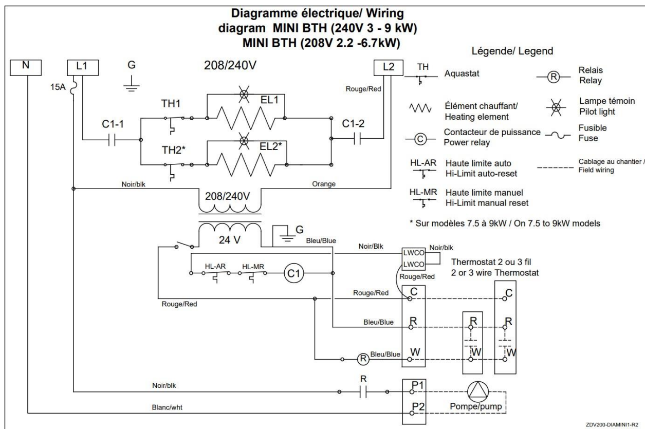
Figure 7 : Diagramme électrique (3-9 KW)
