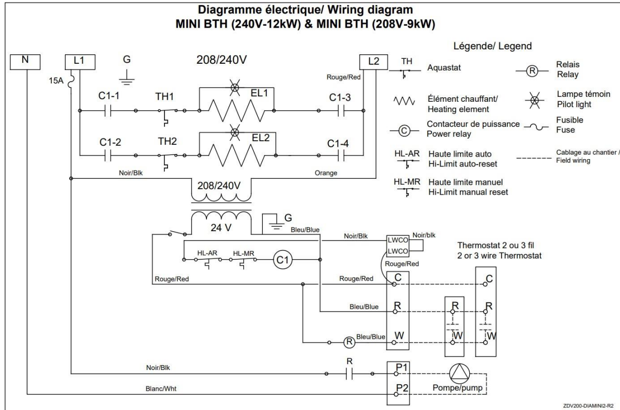
Figure 8 : Diagramme électrique (12 KW)
