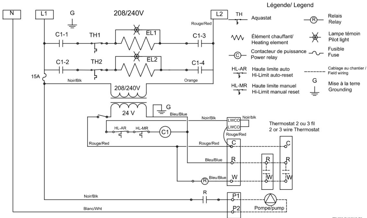
Figure 9 : Diagramme électrique (12 KW)
