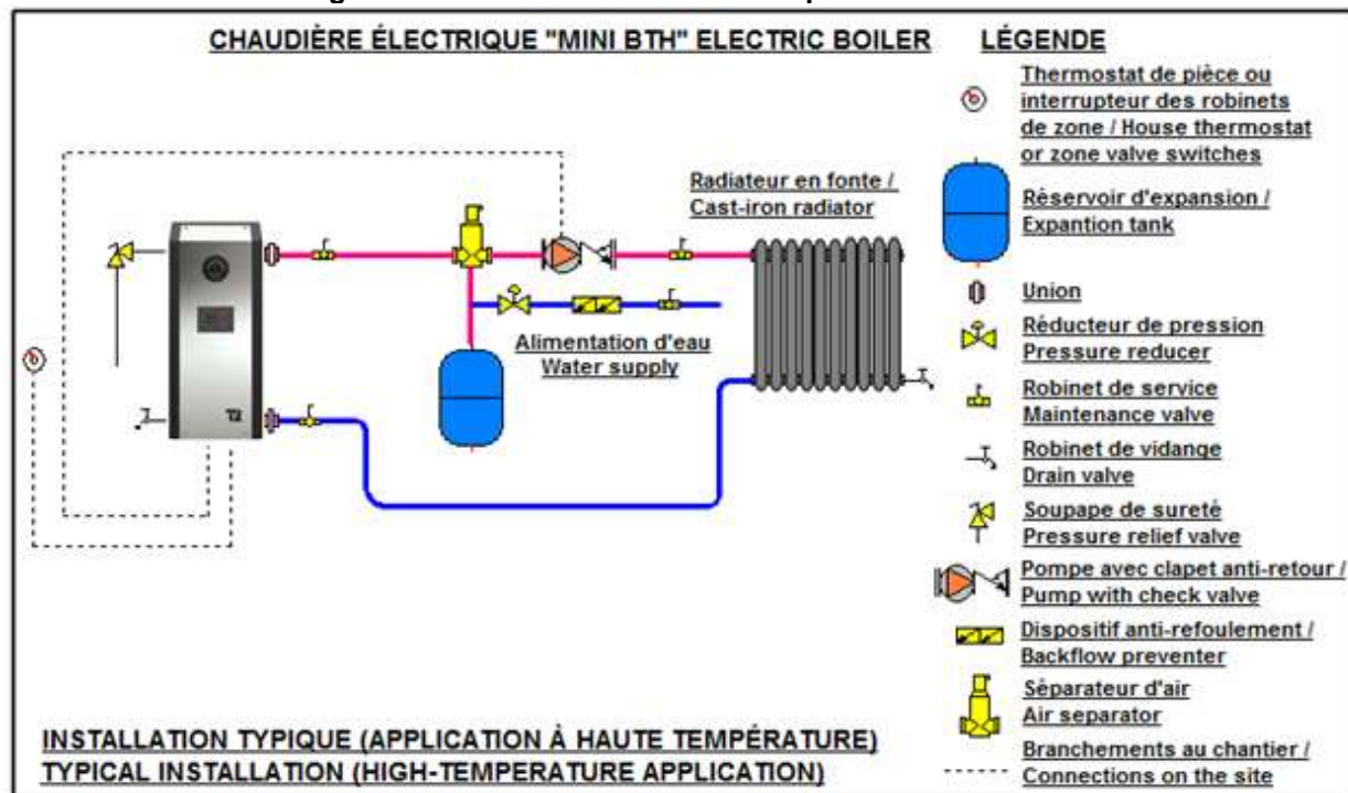
Figure 5 : Schéma d'installation pour applications à haute température
