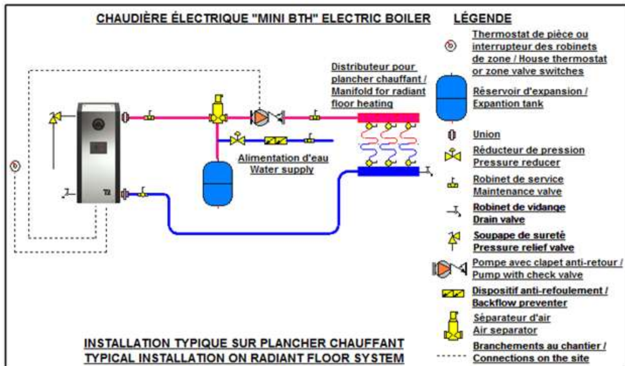
Figure 4 : Schéma d'installation sur plancher chauffant
