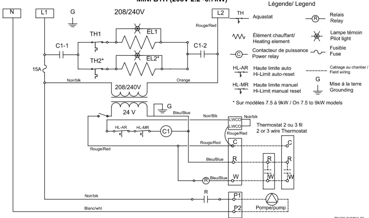
Figure 8 : Diagramme électrique (3-9 KW)
