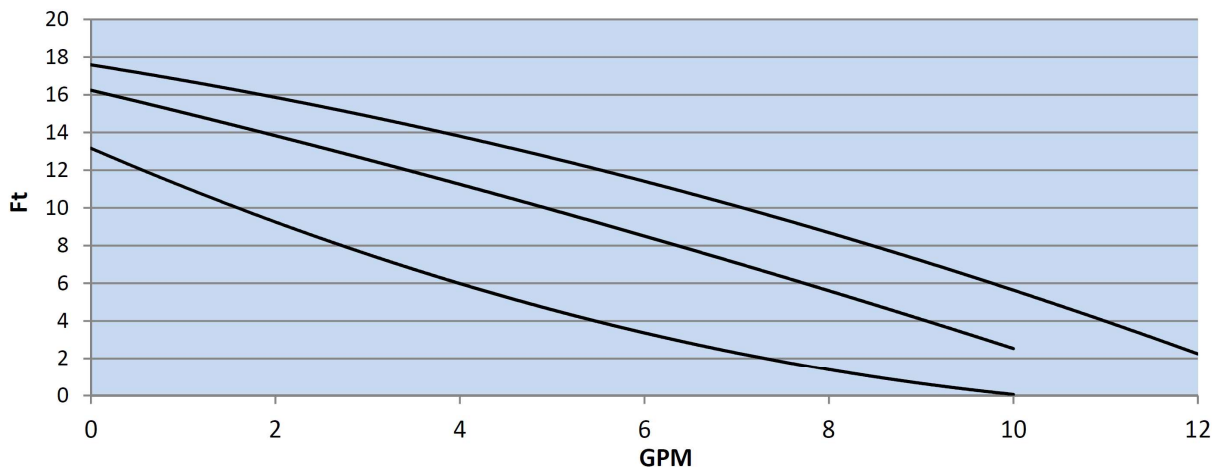
Figure 3 : Performances de la pompe intégrée
