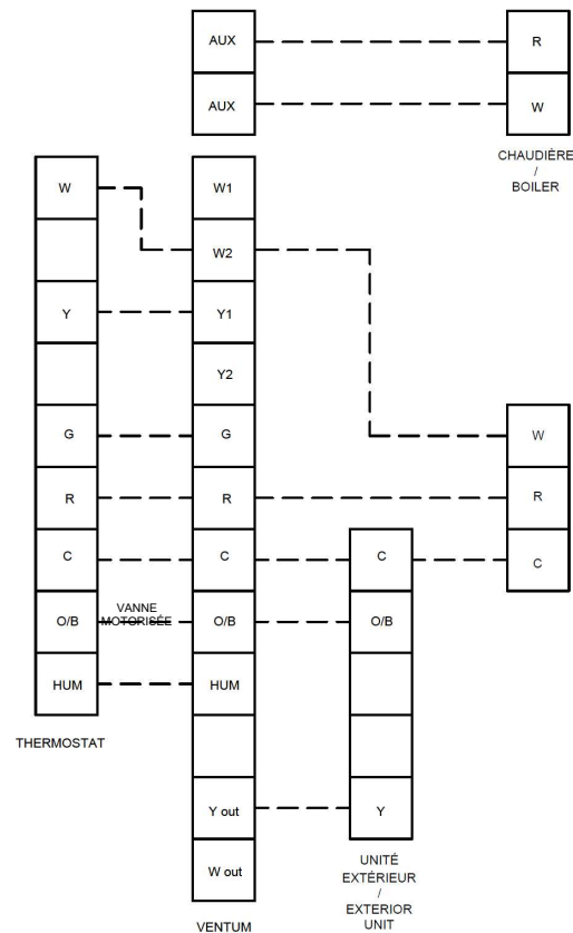
Figure 10 : Exemple de branchement avec thermopompe, chaudière auxiliaire et vanne motorisée
