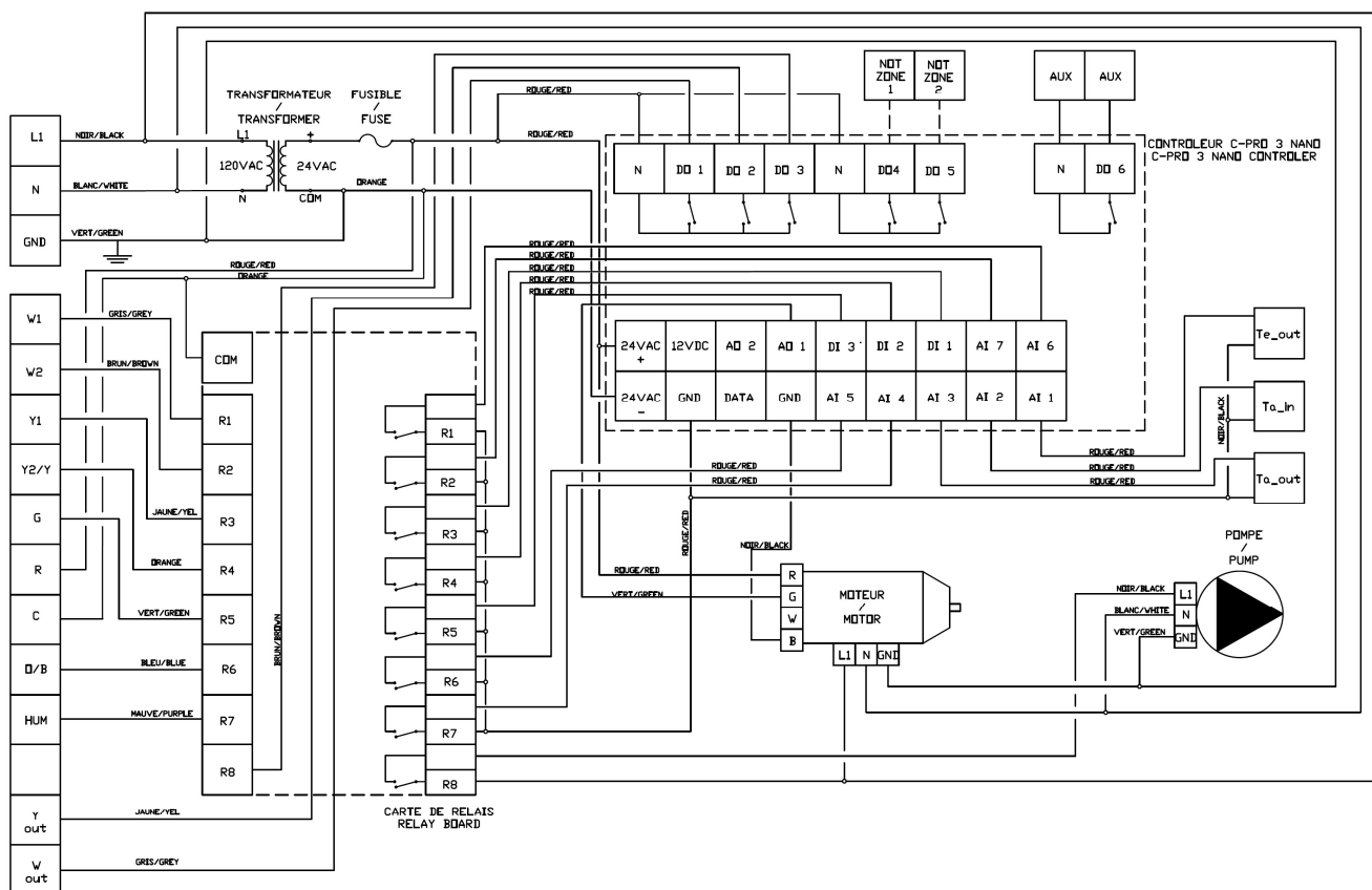
Figure 8 : Schéma électrique avec contrôleur numérique
