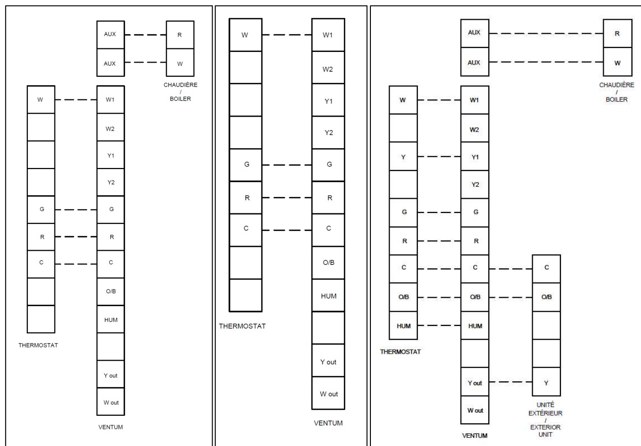
Système avec chaudière seulement et thermostat un stage
