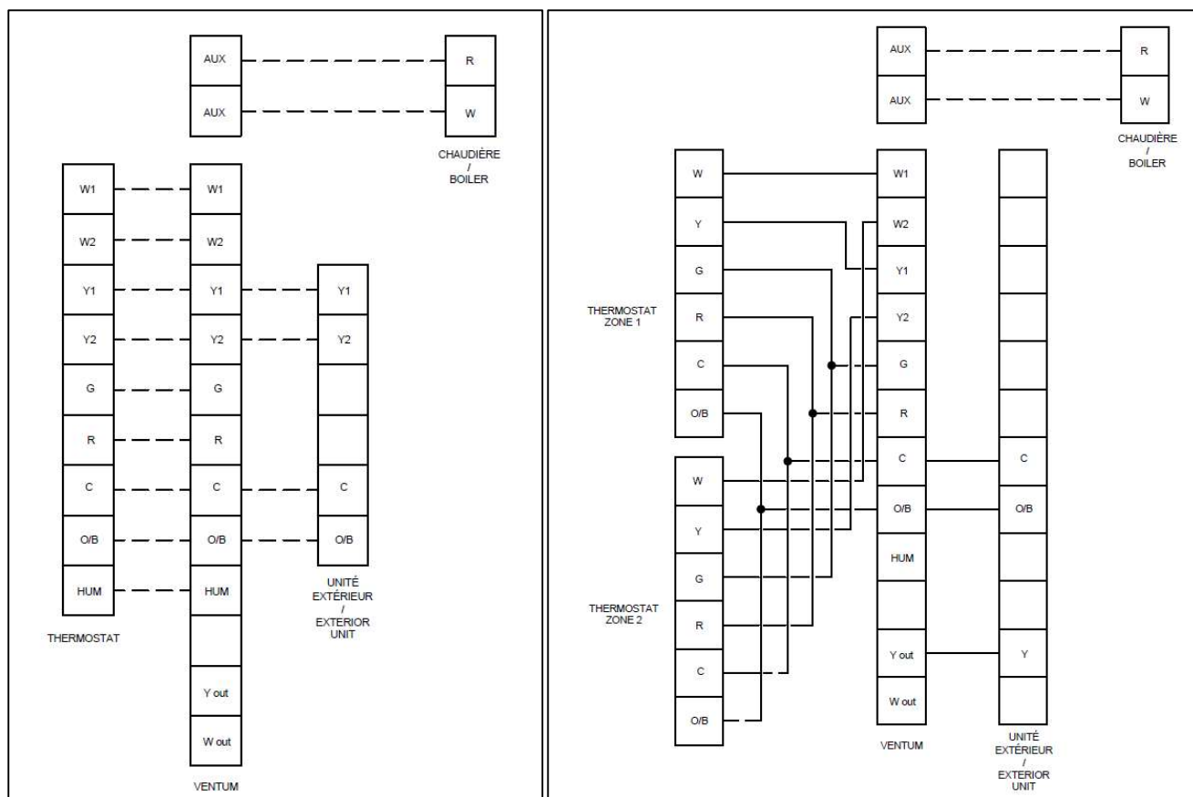
Système avec thermopompe, chaudière en appoint et thermostat deux stages
