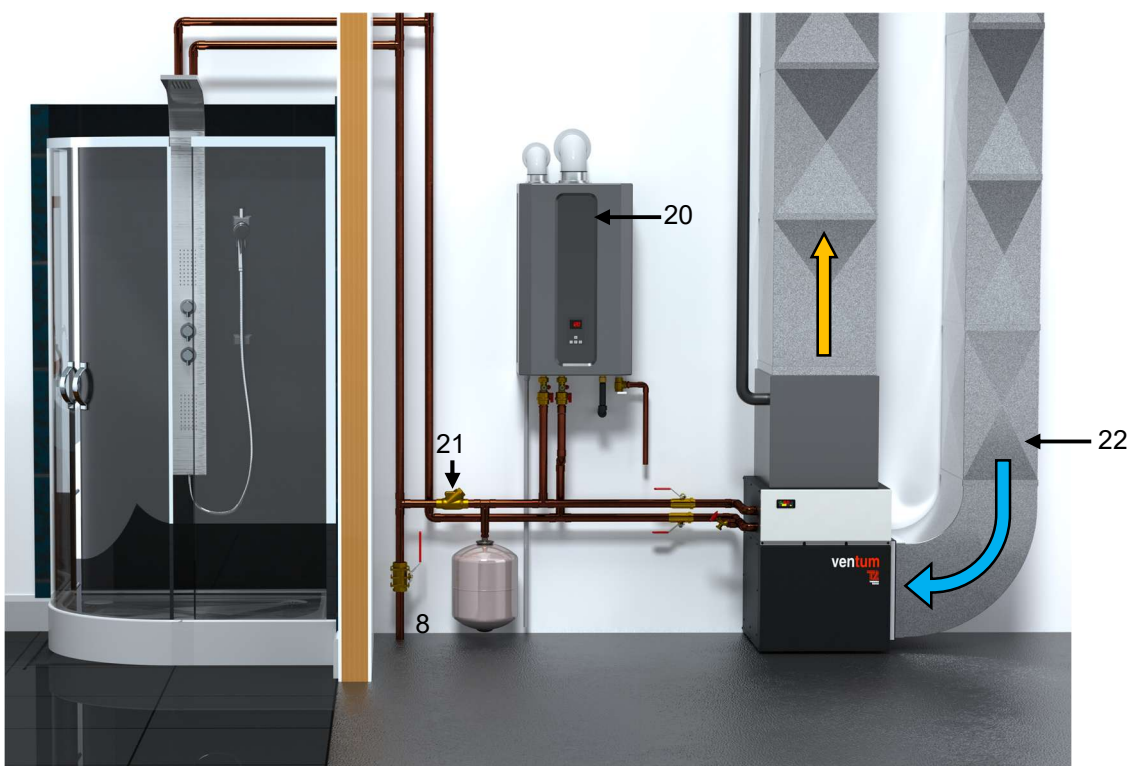
Figure 7 : Installation typique d'un ventilo-convecteur hydronique avec chauffe-eau instantané
