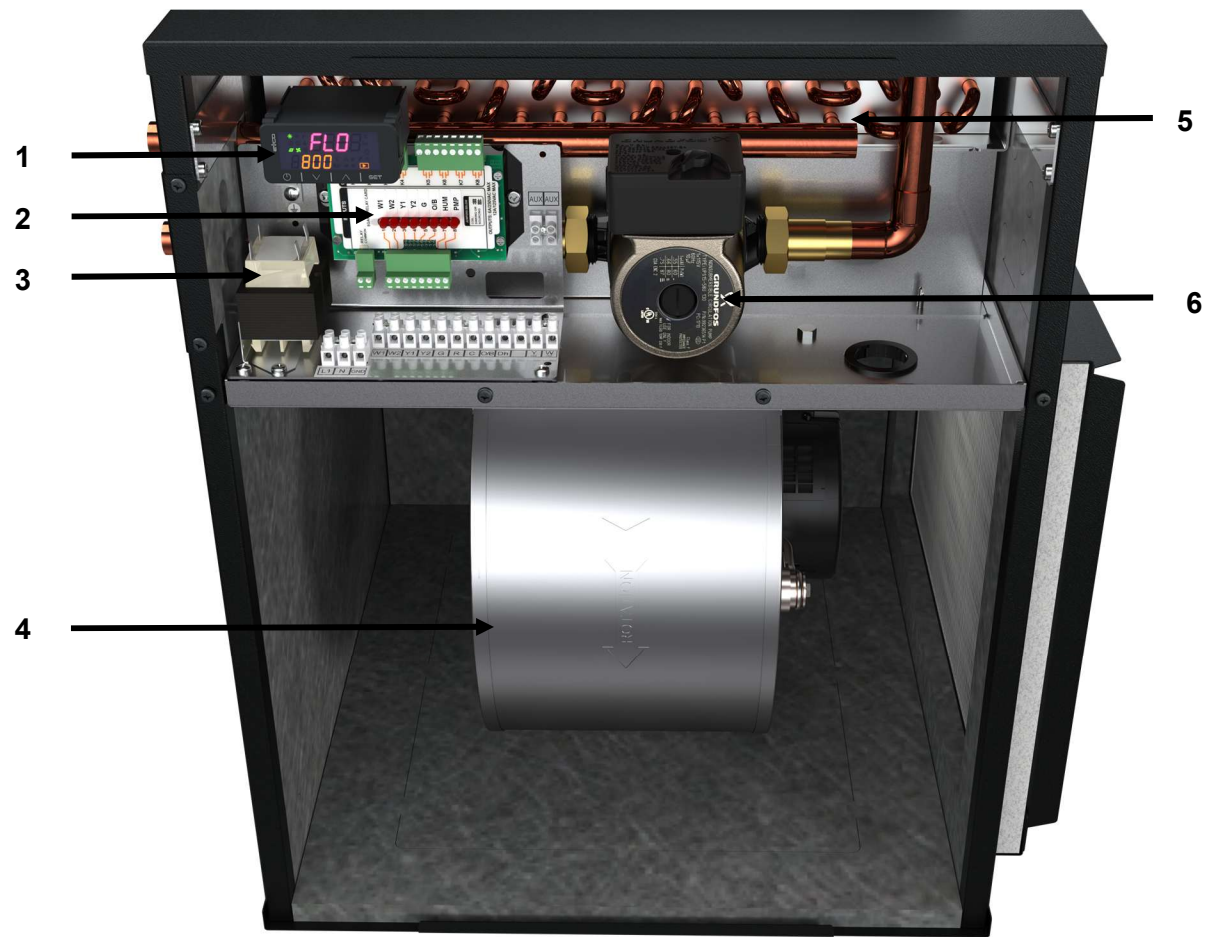
Figure 12 : Vue intérieure du VenTum
