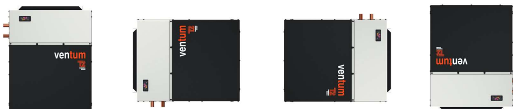
Figure 5 : Positions possibles du ventilo-convecteur hydronique
