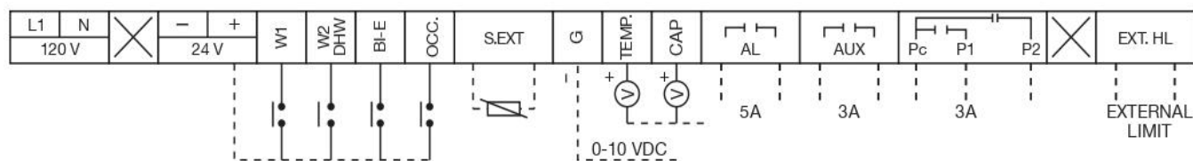
Figure 9 : DIAGRAMME DES RACCORDEMENTS DE CONTRÔLE DE LA CHAUDIÈRE VOLTMAX CONFIGURATION C
