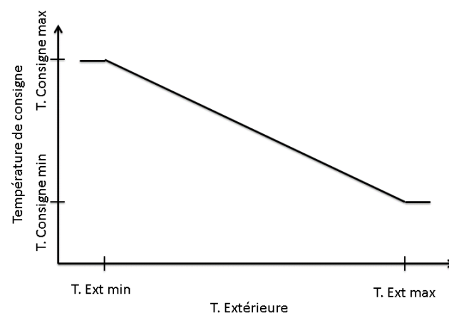
Figure 17 : Courbe d'ajustement Modulation T. Extérieure
